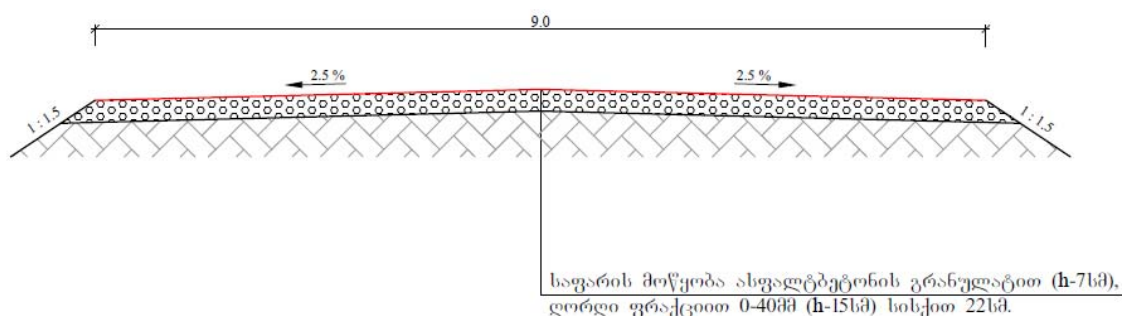
ნახაზი 3.5.1. საპროექტო გზის განივი ჭრილი
