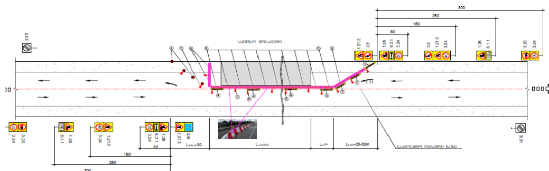
ნახაზი 3.1.1. სამუშაოების პერიოდში სატრანსპორტო ნაკადების რეგულირების პრინციპული სქემა
