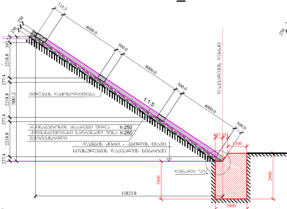
ნახაზი 3.4.1. ნაპირსამაგრი ნაგებობის ჭრილი
