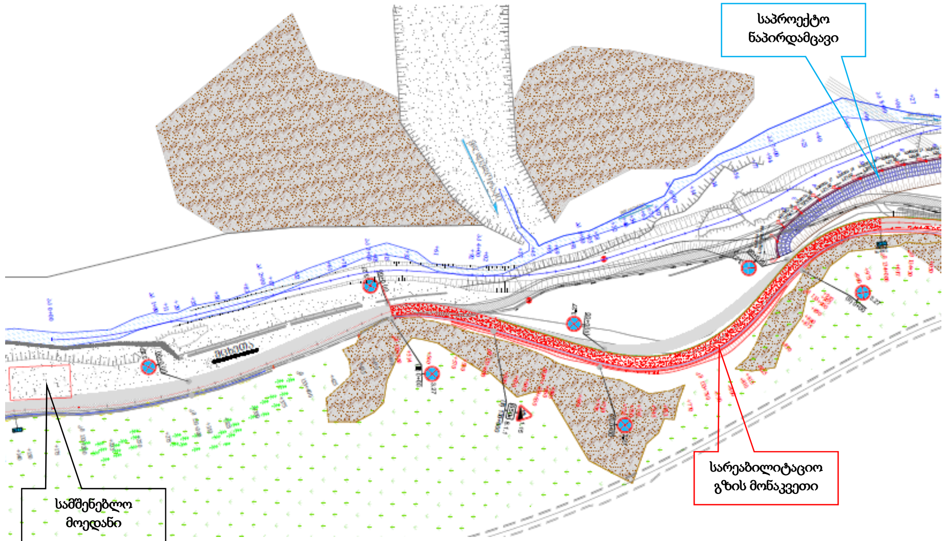
ნახაზი 3.1. პროექტის გენ-გეგმა (ნაწილი 1)
