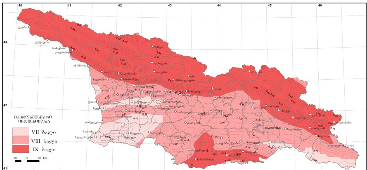
სეისმური საშიშროების რუკა მაქსიმალური კორიზონტული აჩქარება
