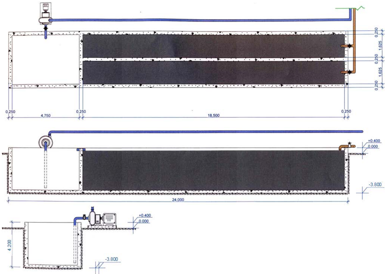
სურათი 3.2.2 სალექარის გეგმა და ჭრილები, მ 1:100
