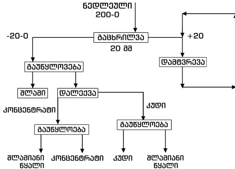
სურათი 3.5.1 გამდიდრების ტექნოლოგიური ციკლი
