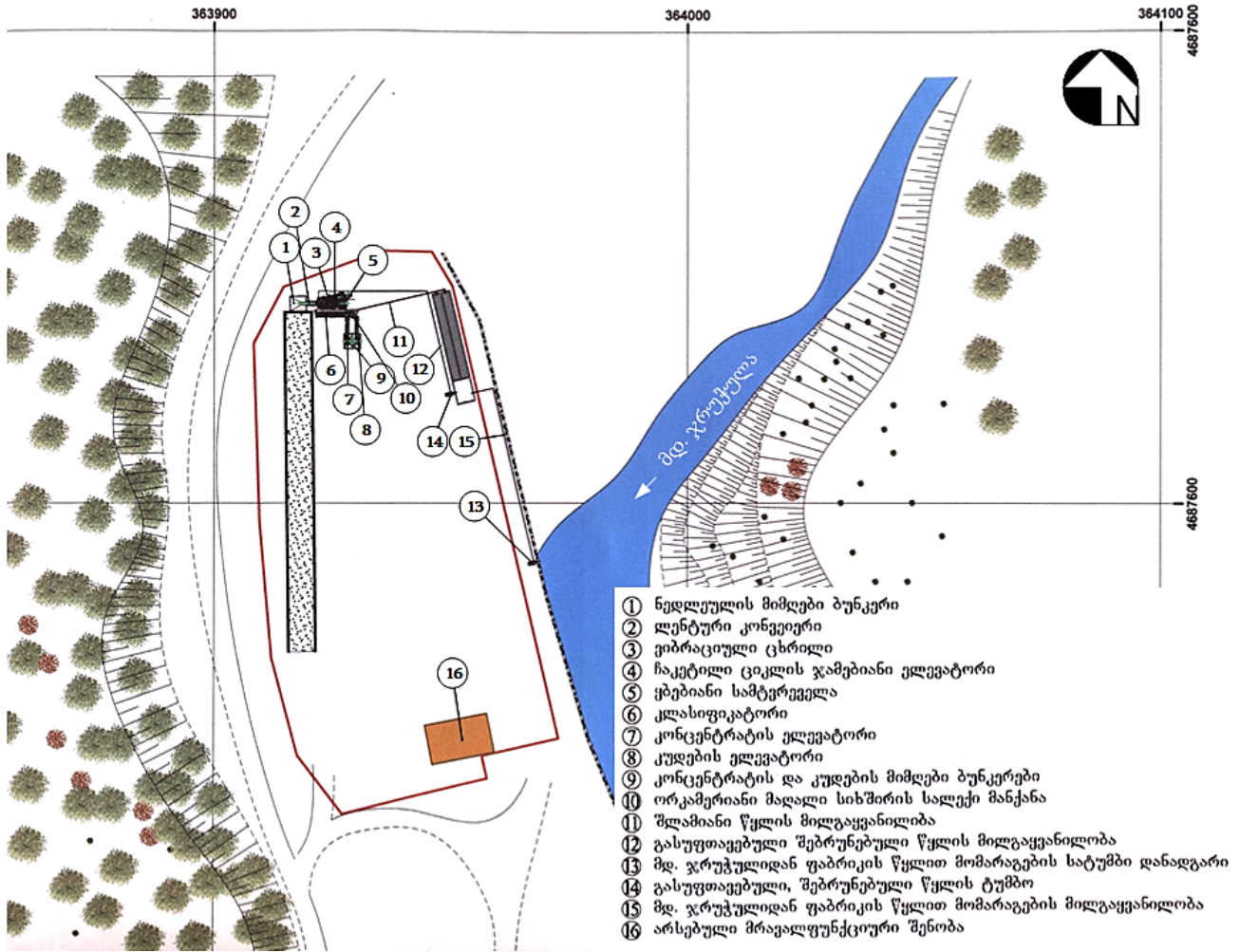
სურათი 3.1.3 საწარმოს გენგეგმა, მ 1:1000
