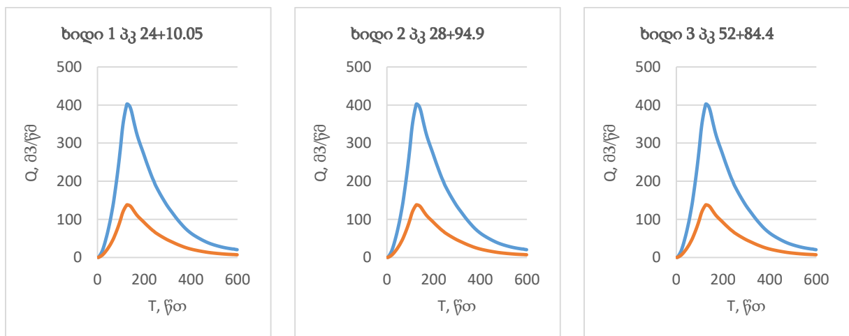
გრაფიკი 5.1 წყლის მაქსიმალური ხარჯის ჰიდროგრაფი და მყარი ნატანის გრაფიკი
