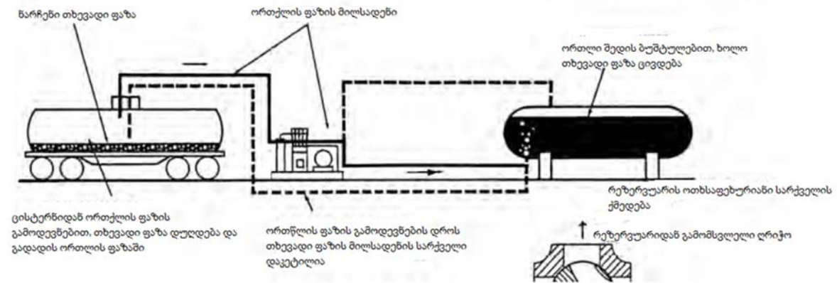
2. ვაკუმისტერნიდან სასაწყობო რეზერვუარში წარჩენი ორთქლის ამოღებისა და გადატარების პროცესი
