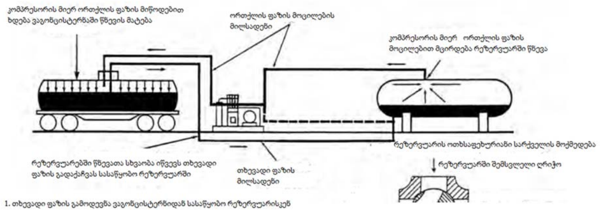
1. თხევადი ფაზის გამოდევნა ვაკუმისტერნიდან სასაწყობო რეზერვუარისკენ
