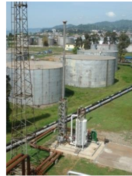
ნახაზი 3.3.1.2. მუქი ნავთობპროდუქტების სამეცროს აირდამჭერი დანადგარი ძირითად ტერიტორიაზე (გ-15) და №№74÷79 რეზერვუარები
