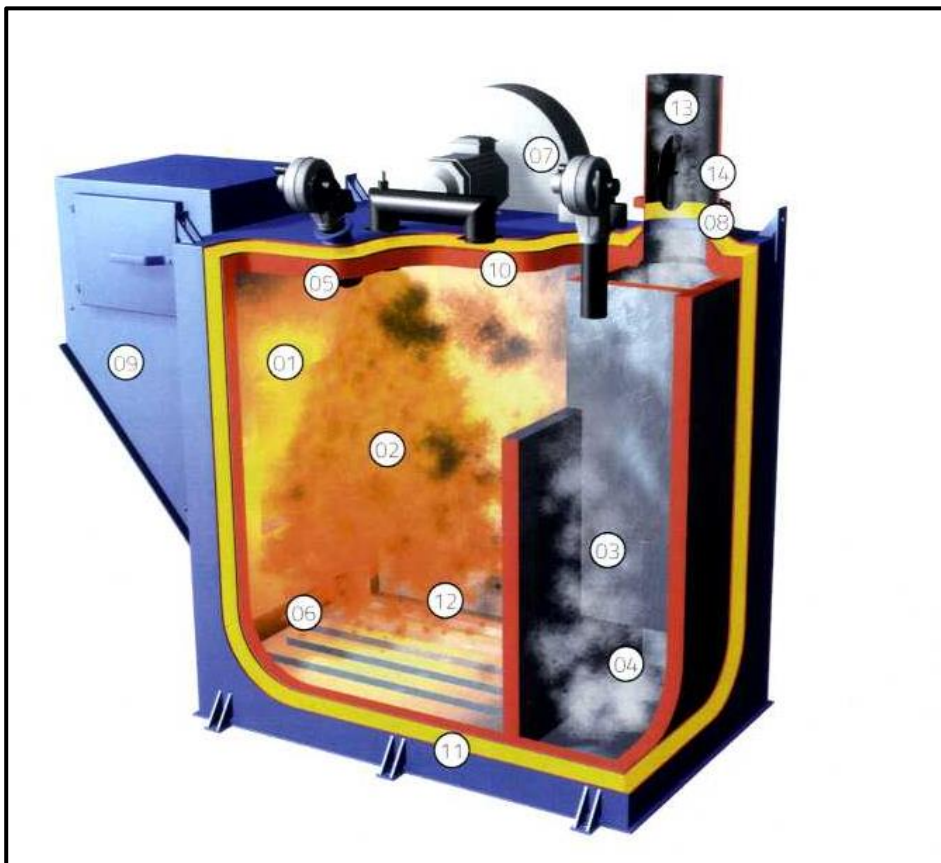
სურათი 3.3.2. ინსინერატორში ნარჩენების წვის სქემა
