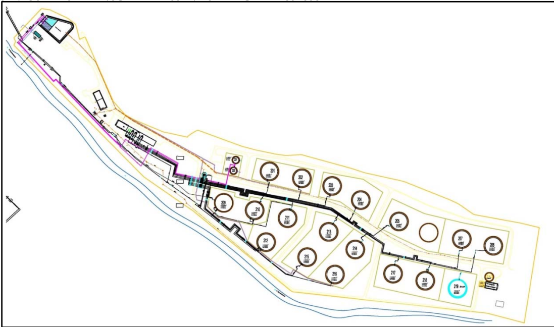
სურათი 1.8.6. შპს „ბათუმის ნავთობტერმინალის“ ნედლი ნავთობის მიღების და შენახვის სადგურის კაპრეშუმის“ (კაპრეშუმის უბნის) გენგეგმა
