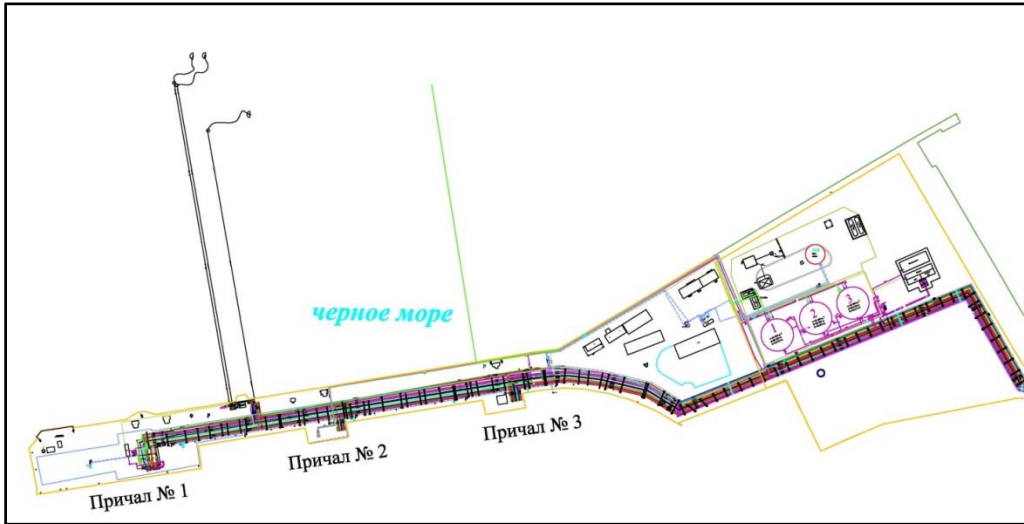
სურათი 2.8.3. შპს „ბათუმის ნავთობტერმინალის ნავთობპროდუქტების საზღვაო ტრანსპორტით მიღების და გადატვირთვის სადგურის (ნავმისადგომების უბნის) ტერიტორიის გენგეგმა
