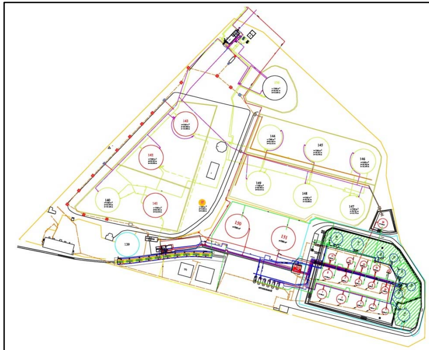
სურათი 1.8.4. შპს „ბათუმის ნავთობტერმინალის ნედლი ნავთობის მიღების და შენახვის სადგურის „ხოლოდნაია სლობოდას“ (ხოლოდნაია სლობოდას უბნის) და იმპორტირებული ნავთობპროდუქტების მიღების და გადატვირთვის საამქროს (ნავთობბაზის უბნის) გენგეგმა
