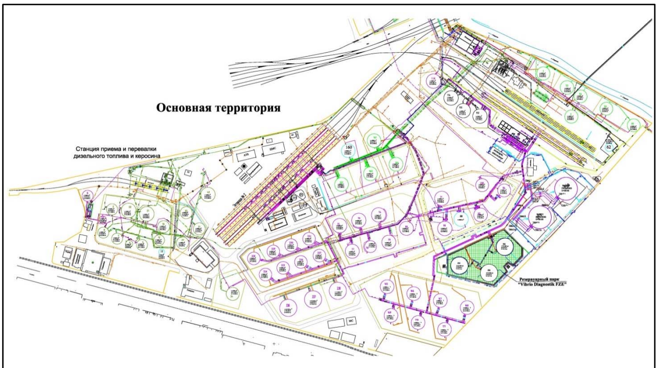
სურათი 1.8.2. შპს „ბათუმის ნავთობტერმინალის ძირითადი ტერიტორიის გენგეგმა
