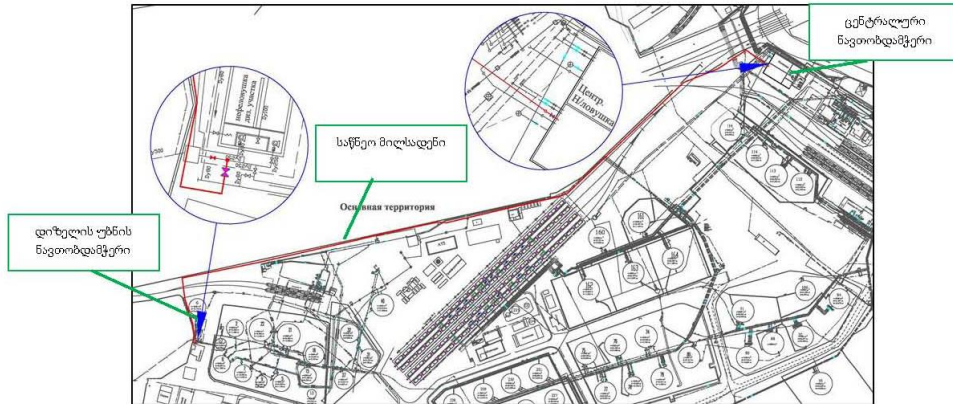
სურათი 3.11.3. დიზელის უბნის ნავთობდამჭერიდან ცენტრალურ ნავთობდამჭერში საწარმოო-სანიაღვრო ჩამდინარე წყლების გამყვანი საწნეო მილსადენის გეგმა
