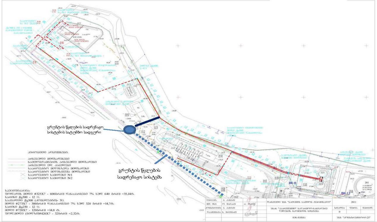
სურათი 3.11.8. კაპრეშვილის უბნის საწარმოო-სანიაღვრო კანალიზაციის სისტემის გეგმა
