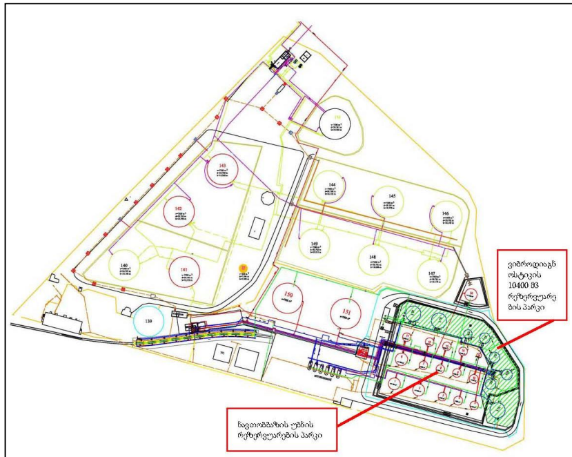
სურათი 3.4.1. ნელი ნათობის მიღების და გადატვირთვის სადგურის „ხოლოდნაია სლობოდას“ რეზერვუარების პარკის გეგმა
