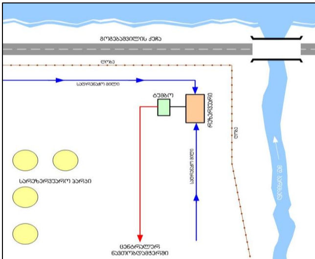
სურათი 3.13.1. გრუნტის წყლების სადრენაჟო სისტემა ნავთის უბანში და სადრენაჟო სისტემის მოწყობის პრინციპული სქემა
