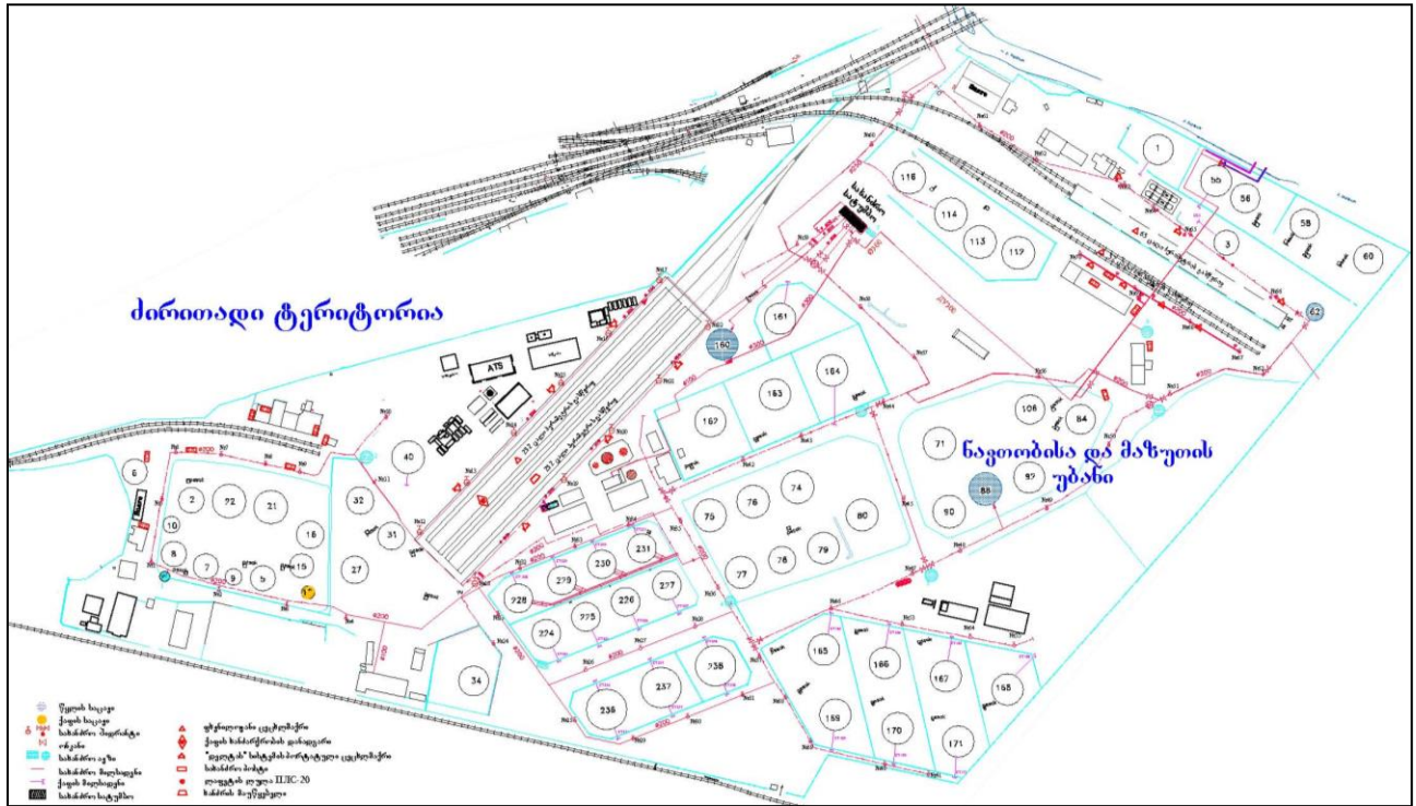
სურათი 4.7.1. ახალი 5000 მ3 რეზერვუარების მშენებლობისთვის დაგეგმილ ტერიტორიაზე სახანძრო-ტექნიკური წყალმომარაგების სისტემის სქემა
