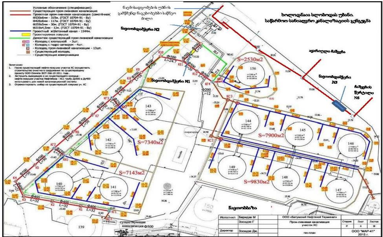
სურათი 3.11.14. N6 საწარმო-სანიადგრო საკანალიზაციო სისტემის გეგმა
