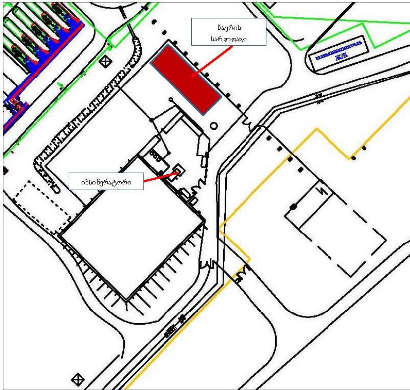
სურათი 3.17.2.1. შპს „სიგმატიკის“ სახიფათო ნარჩენების დამუშავების და გაუვნებლობის (ნავთობშლამების ინსინერაციის) საწარმოს გენგემა.
