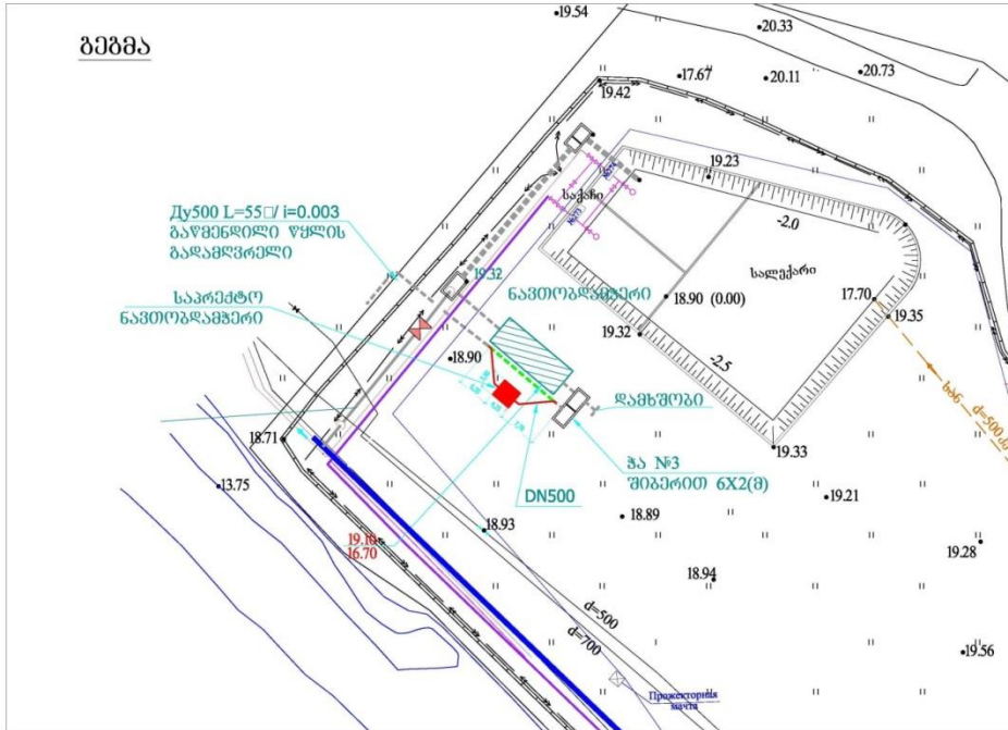
სურათი 3.11.9. კაპრეშვილის უბნის ჩამდინარე წყლების გაწმენდის სისტემის ტექნოლოგიური სქემა.
