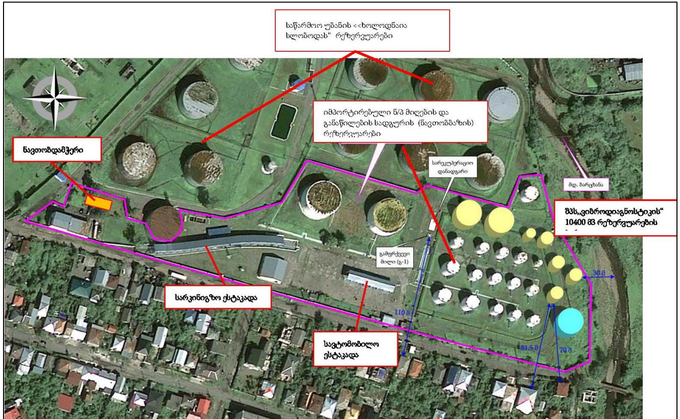
სურათი 3.6.1. იმპორტირებული ნავთობპროდუქტების მიღების და განაწილების სამუქროს და Vibro Diagnostik FZE-ს (ფერადი) სარეზერვუარო პარკები
