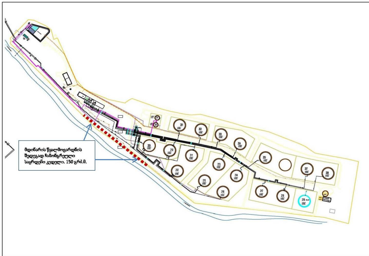
სურათი 3.5.1. ნედლი ნავთობის მიღების და გადატვირთვის სადგურის „კაპრემუმის“ რეზერვუარების პარკის სიტუაციური გეგმა
