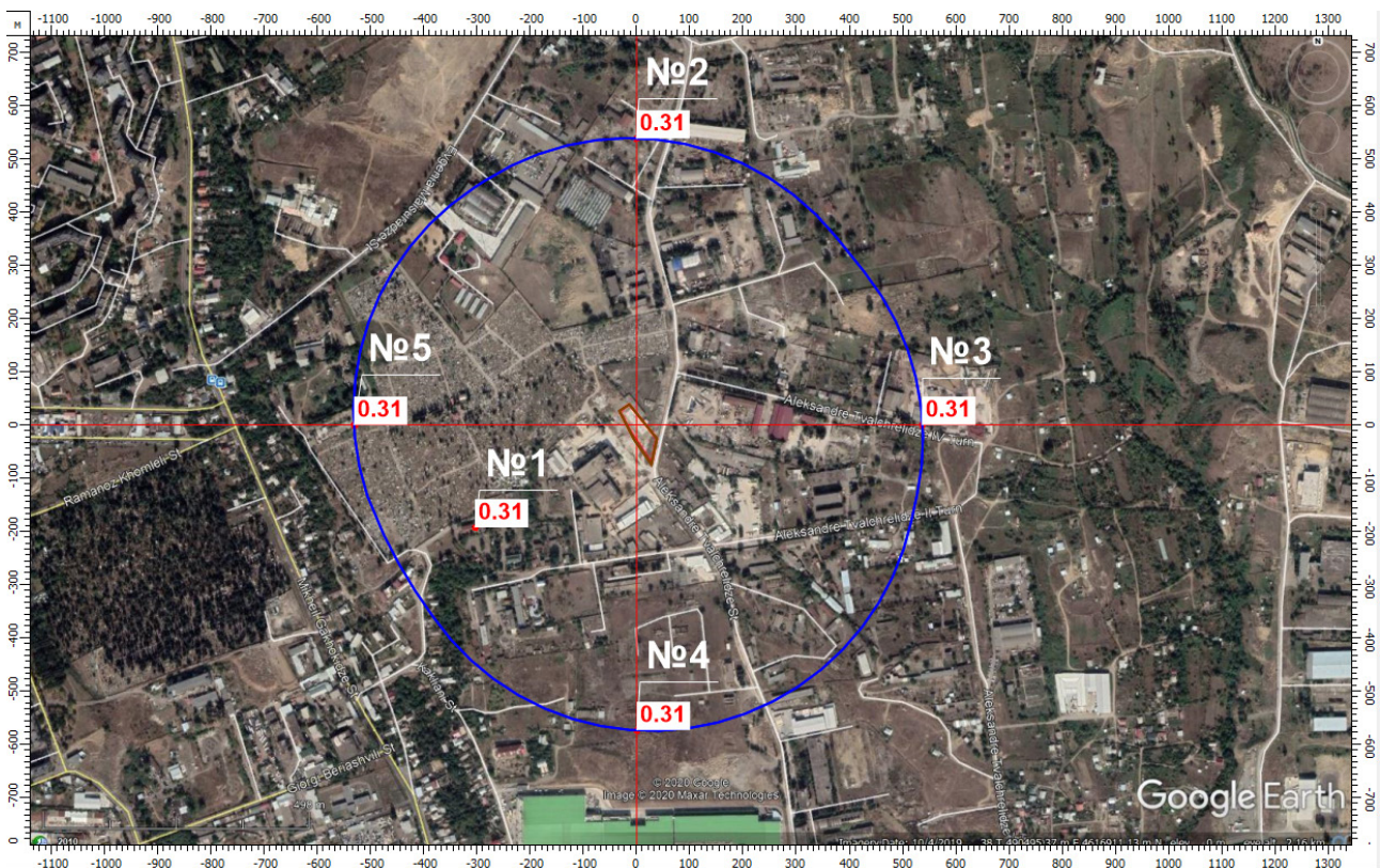
ნივთიერება: 0337 ნახშირბადის ოქსიდი. მაქსიმალური კონცენტრაციები უახლოეს დასახლებასთან (წერტ. N1) და ნორმირებული 500მ. ზონის სზალვარზე (წერტ. N 2-5).
