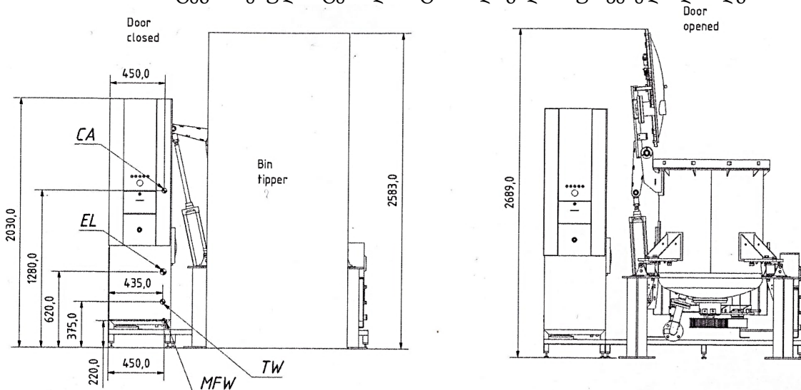
ნახაზი 3.4.3. Celitron-ის ინტეგრირებული სტერილიზატორი და გადამამუშავებელი დანადგარის ზომები
