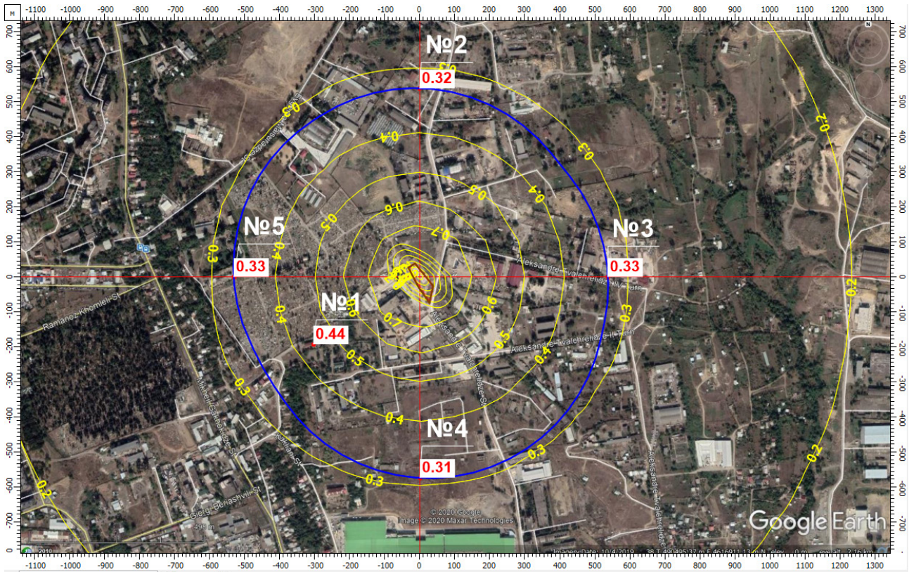
ნივთიერება: 0301 აზოტის დიოქსიდი (აზოტის (IV) ოქსიდი). მაქსიმალური კონცენტრაციები უახლოეს დასახლებასთან (წერტ. N1) და ნორმირებული 500მ. ზონის სზაღვარზე (წერტ. N 2-5).
