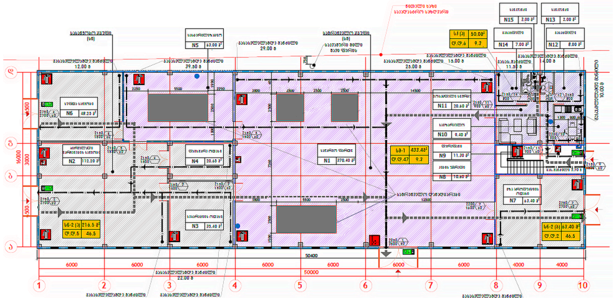
ნახაზი 4.3.3. საწარმოო შენობის გეგმა ხანძარსაწინააღმდეგო ინვენტარის განლაგების დატანით, მ 1:100
