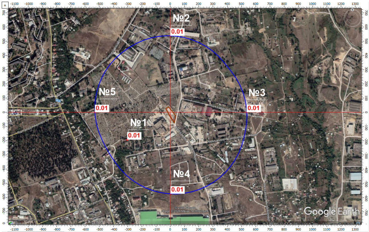
ნივთიერება: 0328 ნახშირბადი (ჭვარტლი). მაქსიმალური კონცენტრაციები უახლოეს დასახლებასთან (წერტ. N1) და ნორმირებული 500მ. ზონის სზალვარზე (წერტ. N 2-5).
