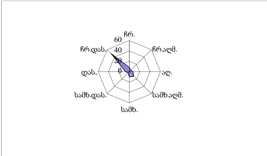
ნახ. 2.1 ქარის მიმართულებების განმეორადობა (პროცენტებში)
