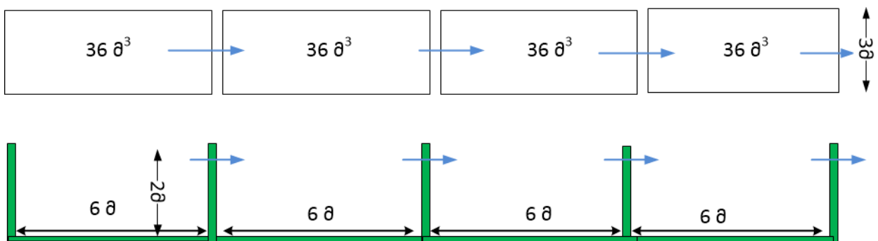
ნახაზი 4.2.1.2 სალექარის გეგმა და ჭრილი
