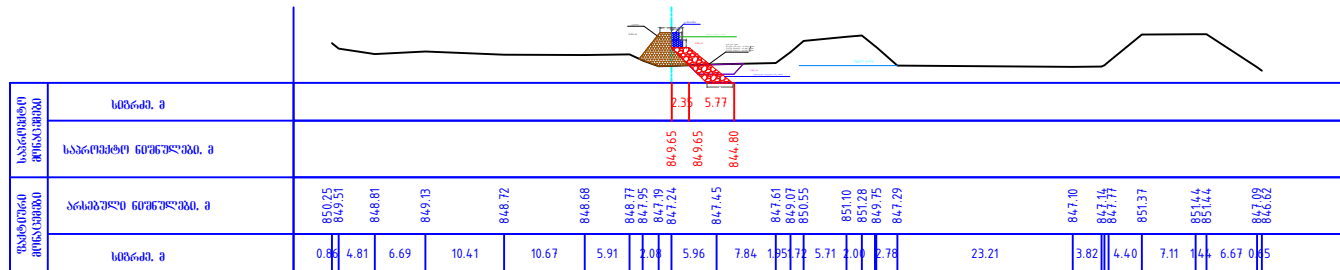
განივი პროფილი ПК 1+20.00
