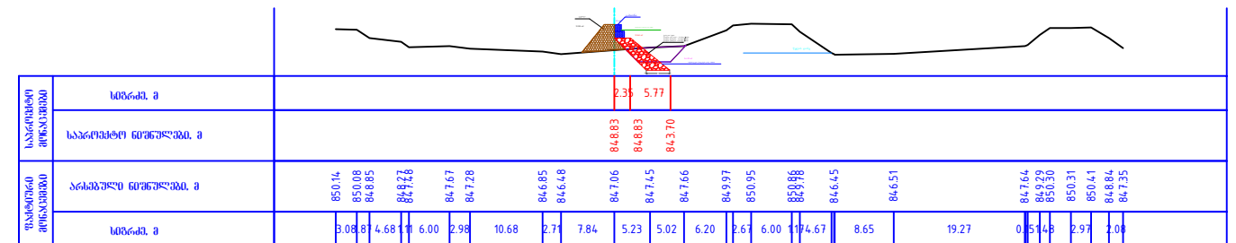
განივი პროფილი ПК 1+80.00
