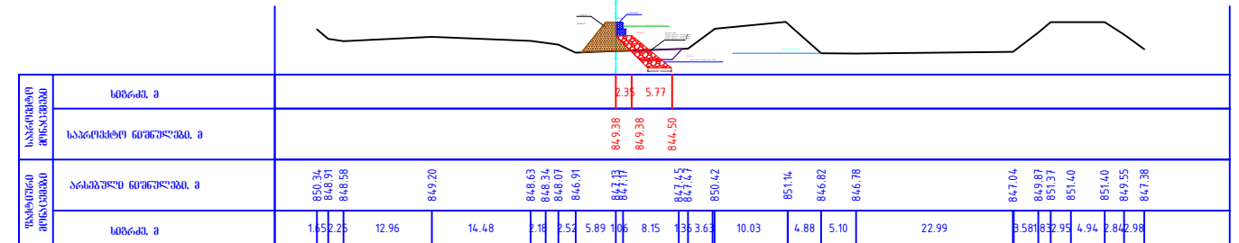
განივი პროფილი ПК 1+40.00
