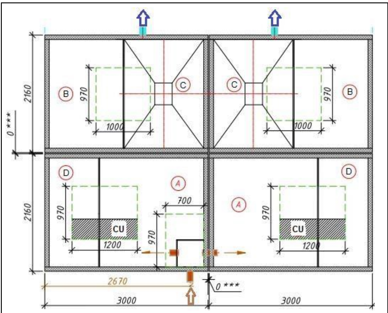
ნახაზი 2.3.6.1. გამწმენდი ნაგებობის სქემა
