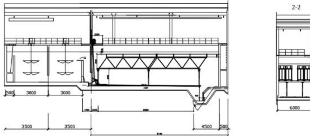
საპროექტო სალექარი და სარეაგენტო 1-1
