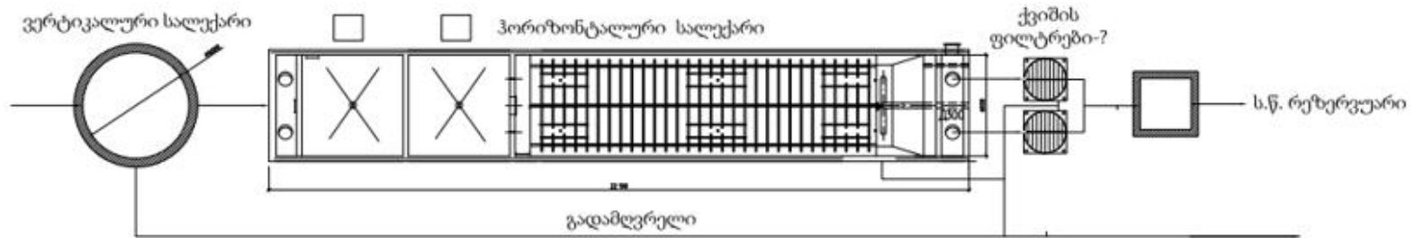
ტექნოლოგიური სქემა 18 ლ/წმ
