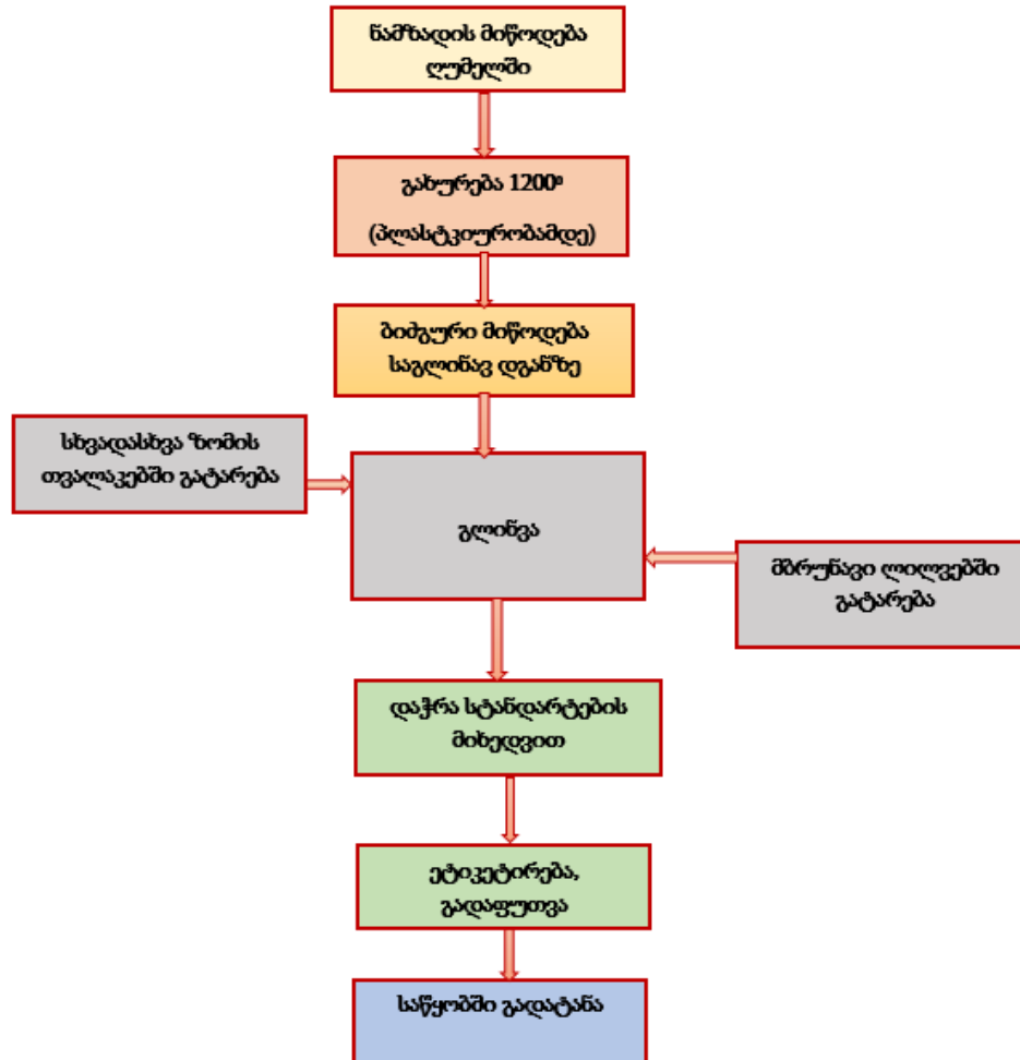
ნახაზი 3.3. გლინვის ტექნოლოგიური სქემა
