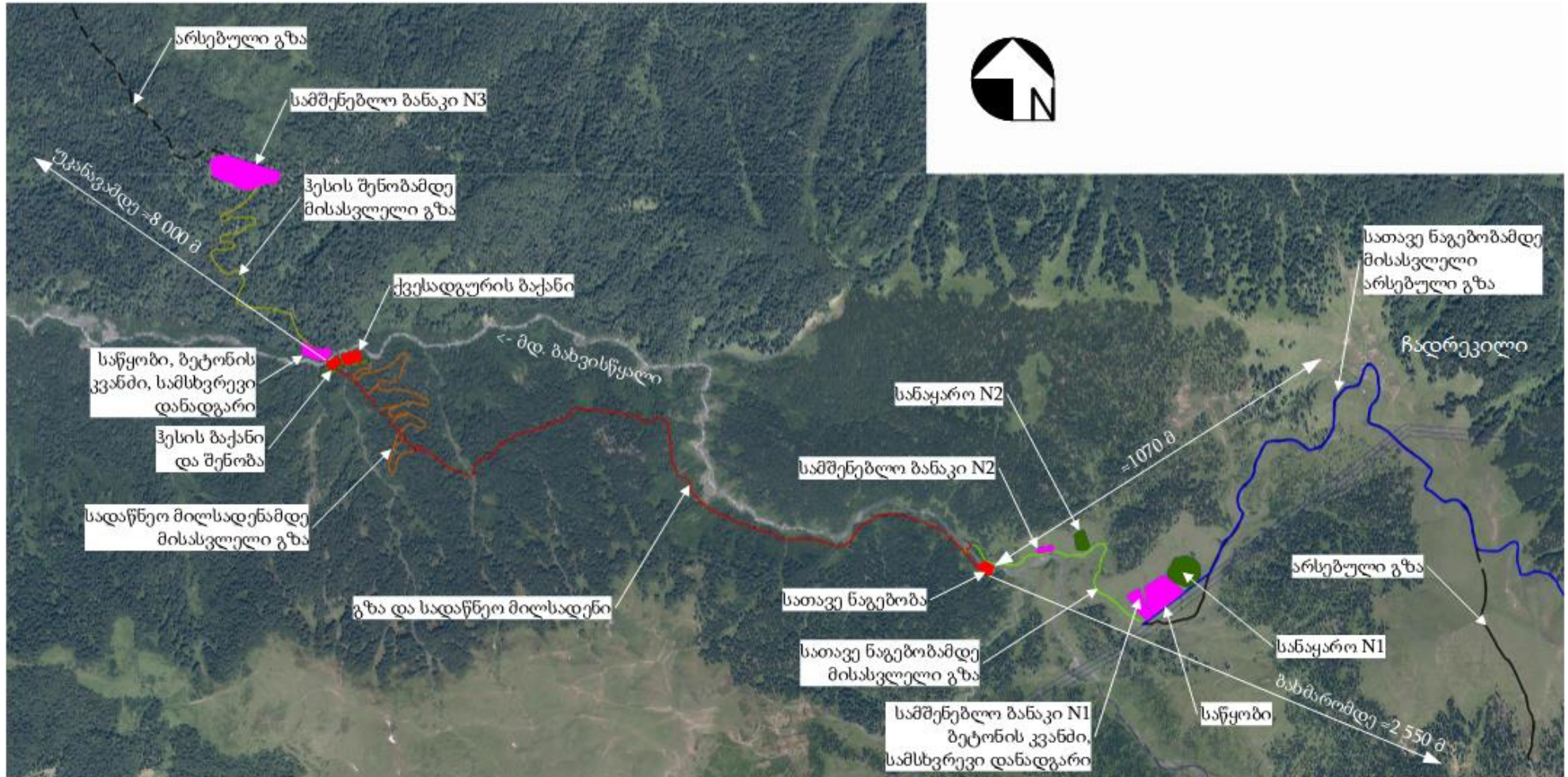
ბაზვი 1 ჰესის კომუნიკაციების განლაგების სიტუაციური სქემა
