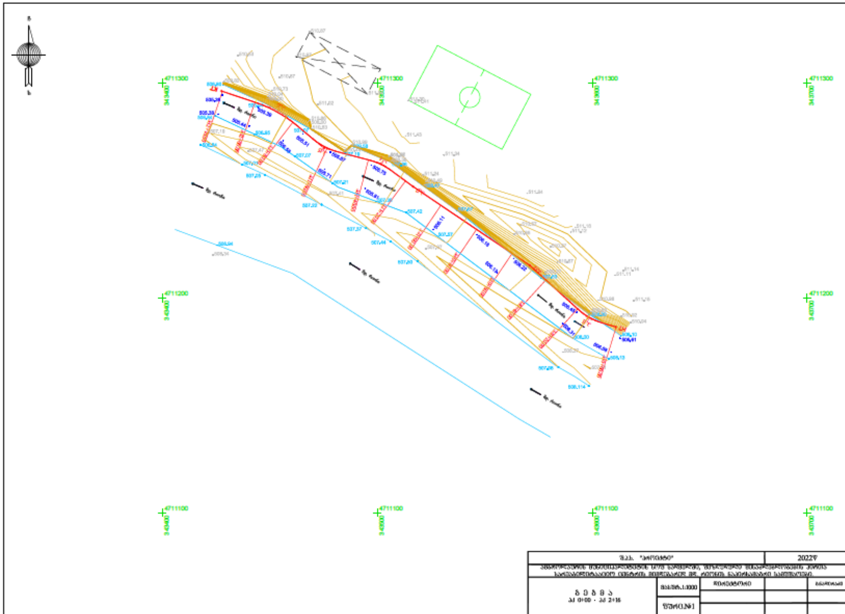
ნახაზები 3.1. პროექტის გენ-გეგმა
