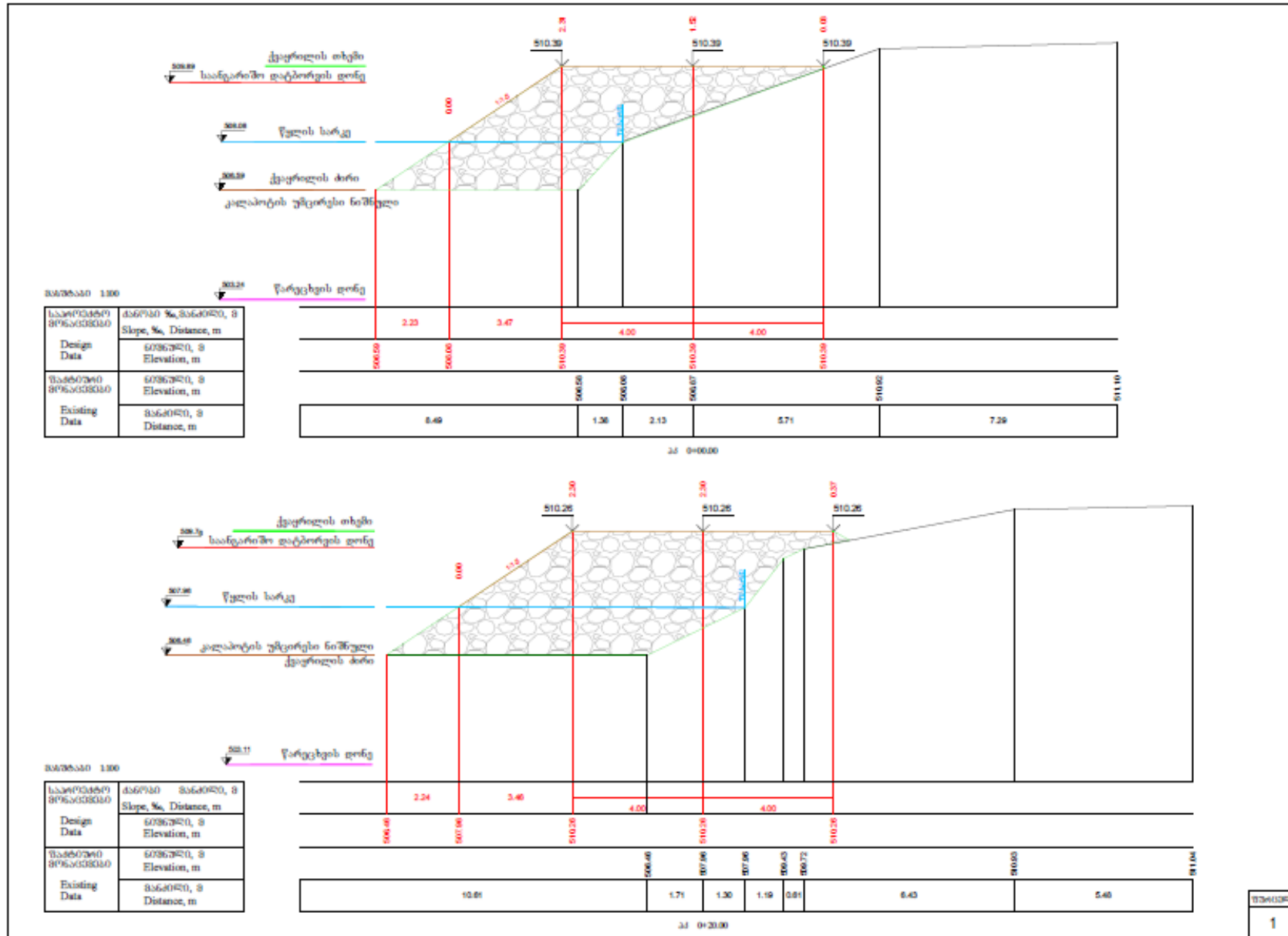
ნახაზები 3.3. ნაპირდამცავი ნაგებობების ტიპური განივი ჭრილი
