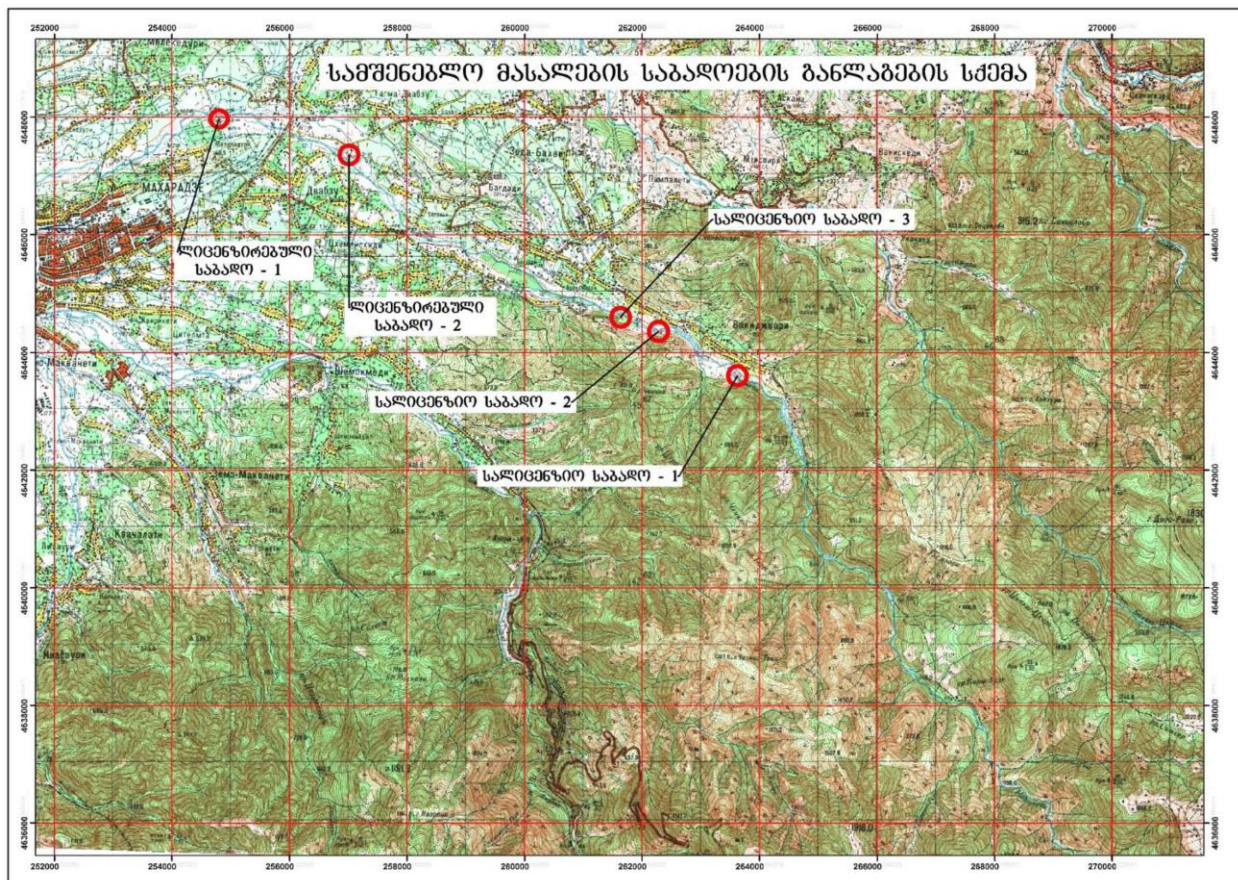
სურათი 1 სამშენებლო მასალების საბადოების განლაგების სქემა
