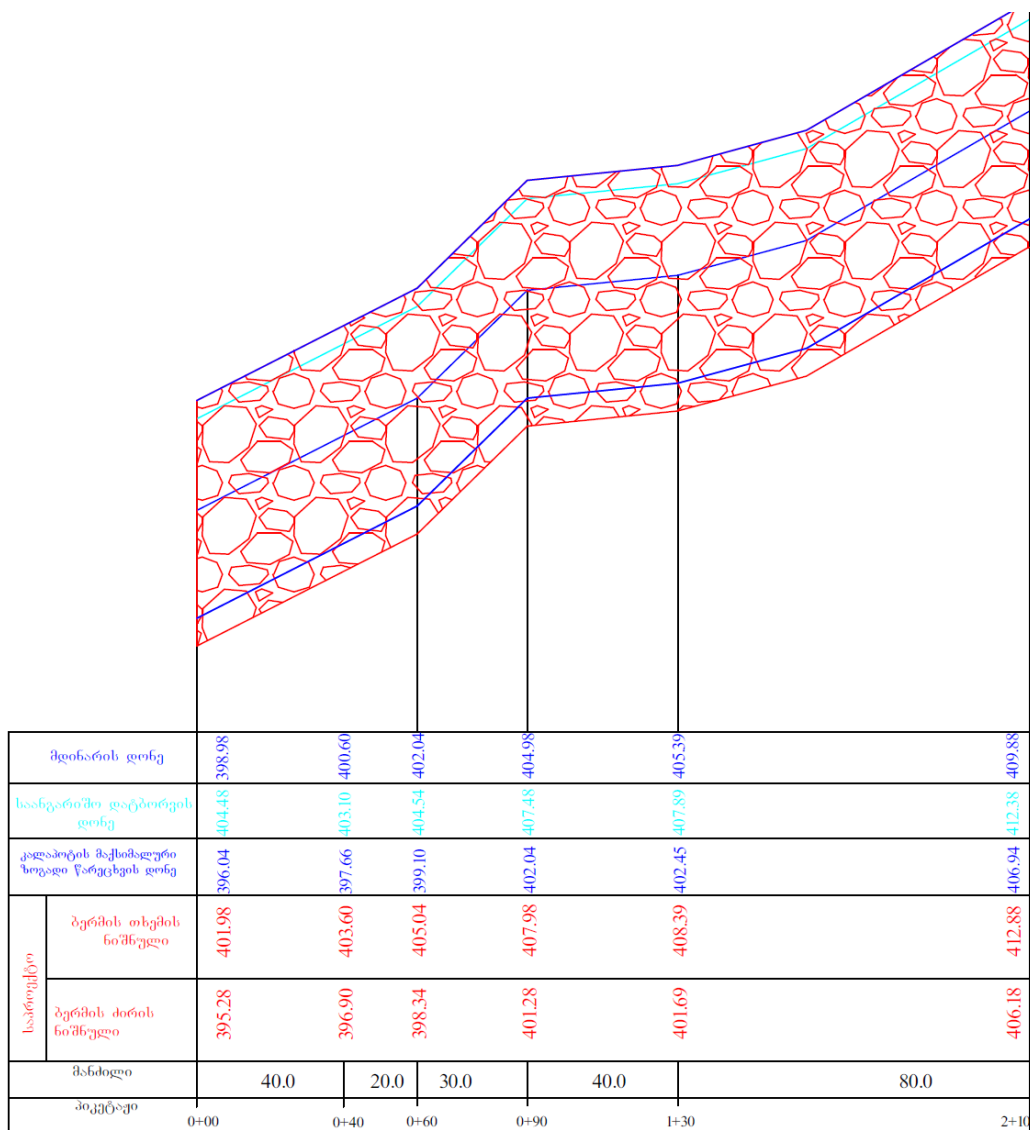
ნახაზი 4 ნაპირსამაგრი კედლის გრძივი კვეთი
