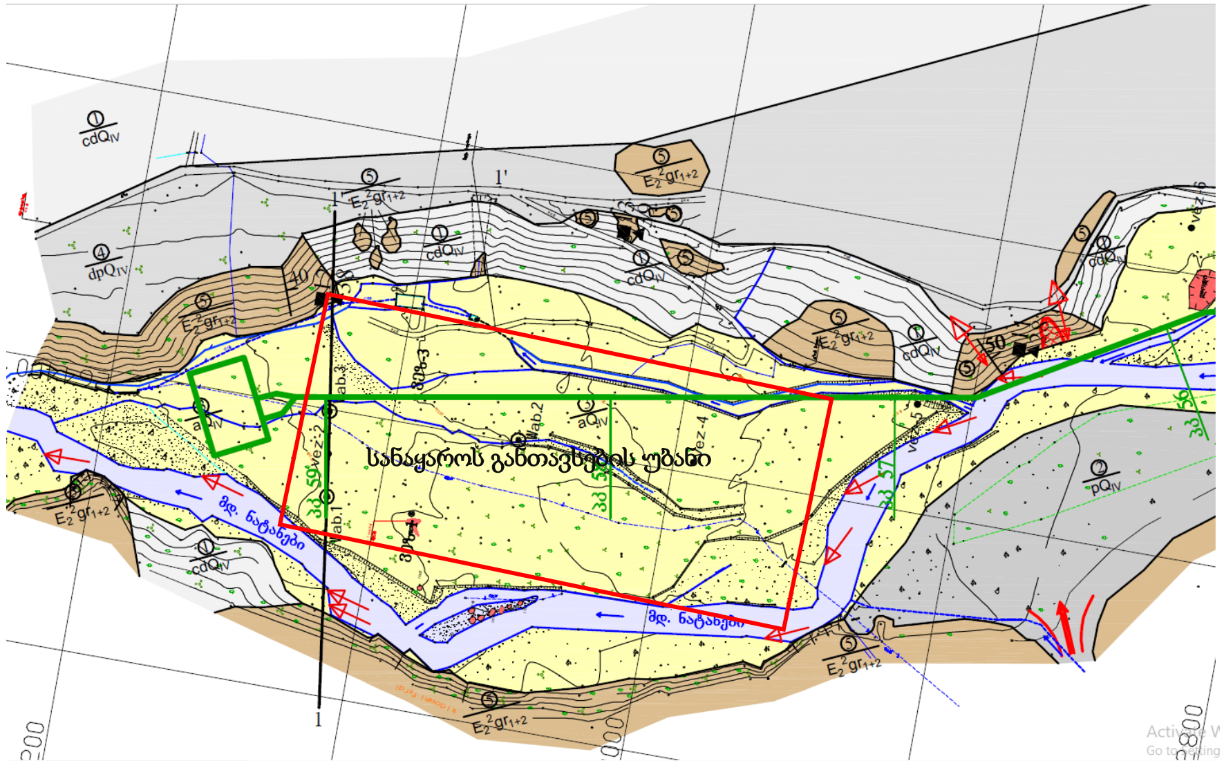
ნახაზი 7 საკვლევი უბნის გეოლოგიური რუკა
