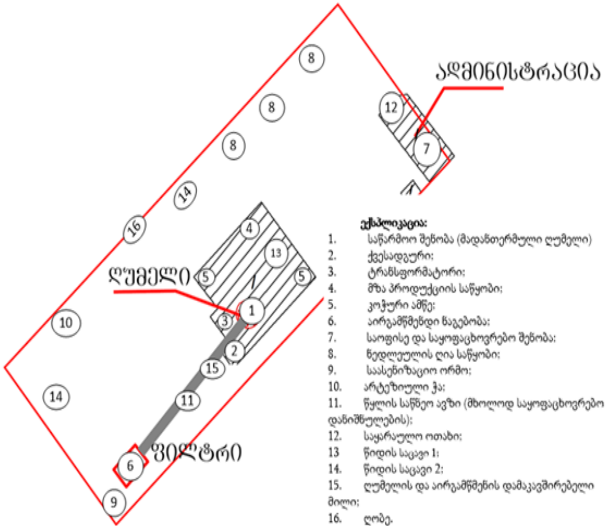
ნახაზი 1 საწარმოს გენ-გეგმა
