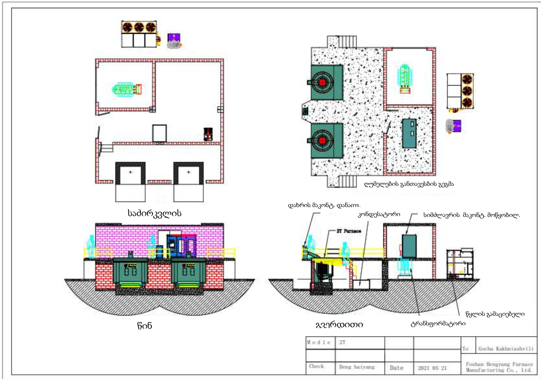
ნახ.8.2. ინდუქციური ღუმელების და სხვა დამხმარე დანადგარების მოწყობის სქემა.
