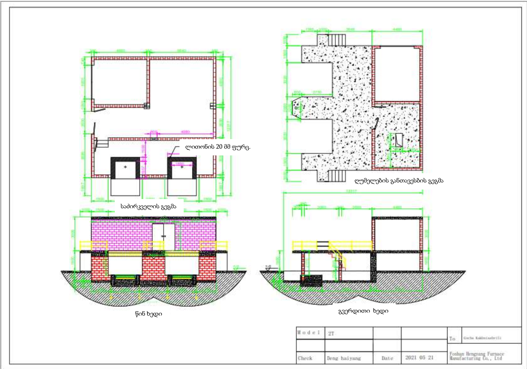
ნახ.8.1. ინდუსტრიული ღუმელის მოწყობის სქემა
