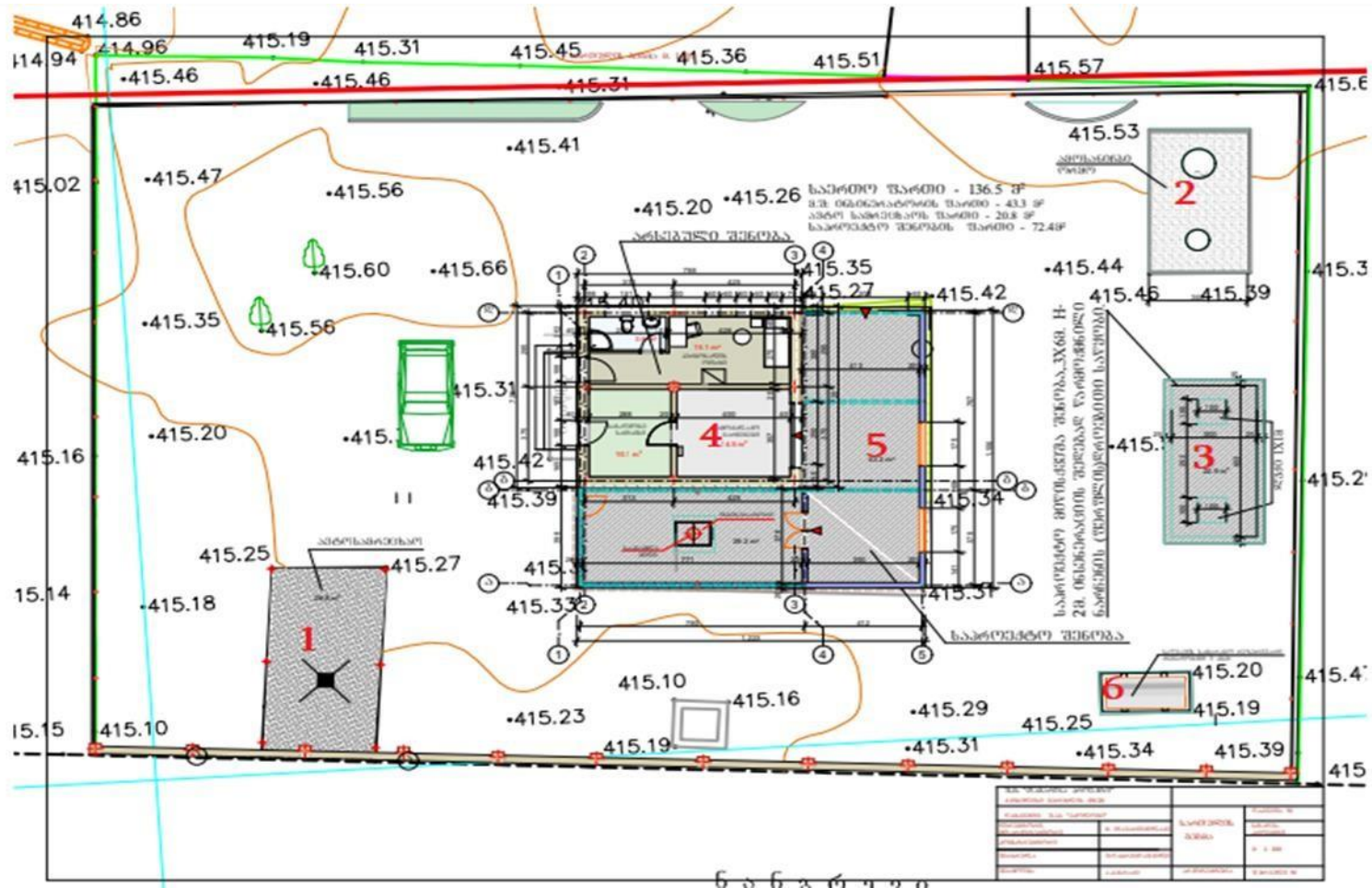
ფიგურა 2.4 საწამოს გენ-გეგმა ექსპლიკაციით
