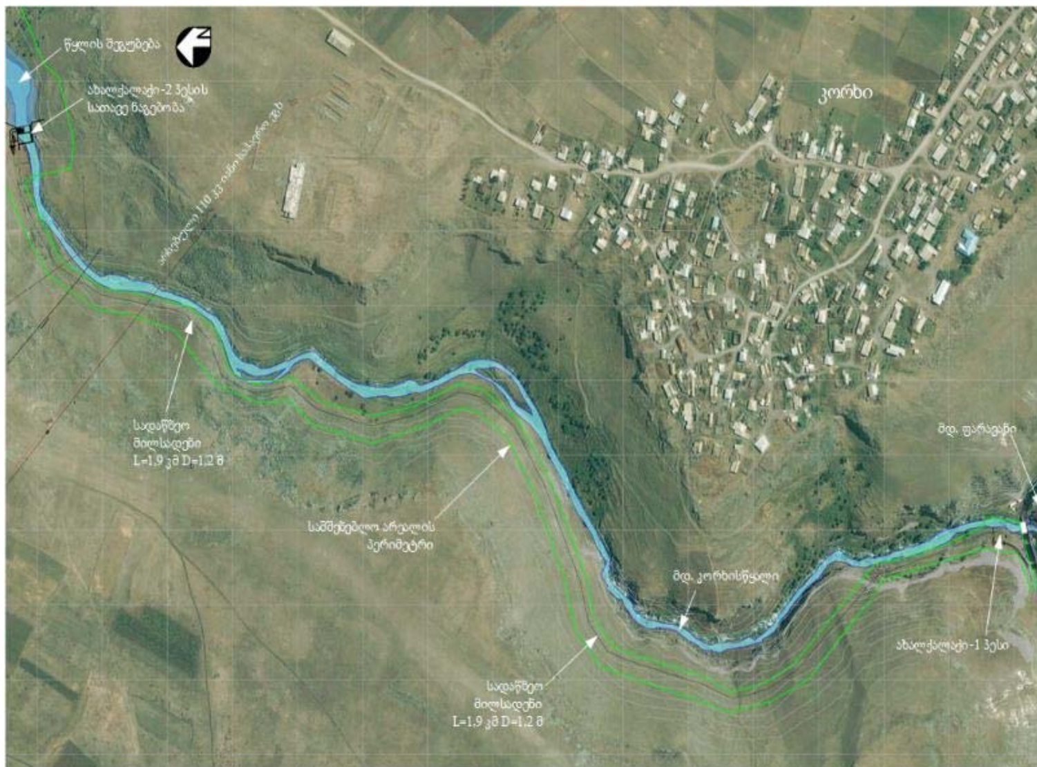
ნახაზი 2.2.3 ახალქალაქი 2 ჰესის გენგეგმა
