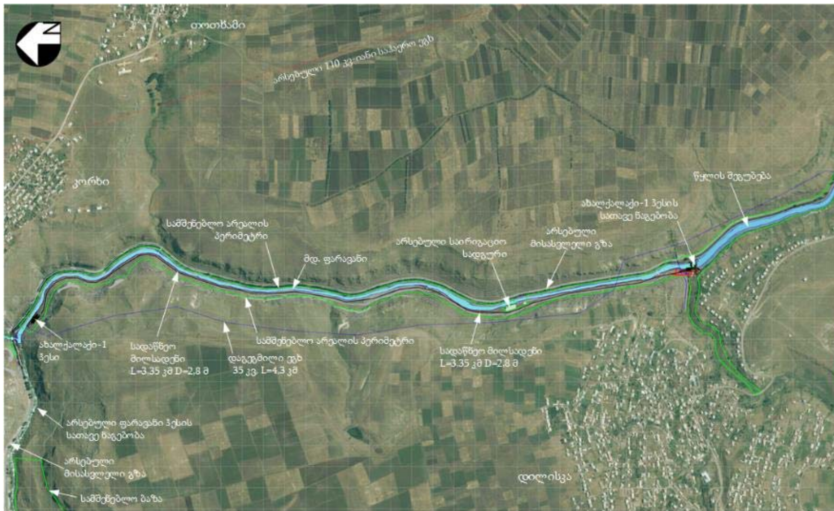
ნახაზი 2.2.2 ახალქალაქი 1 ჰესის გენერალური გეგმა
