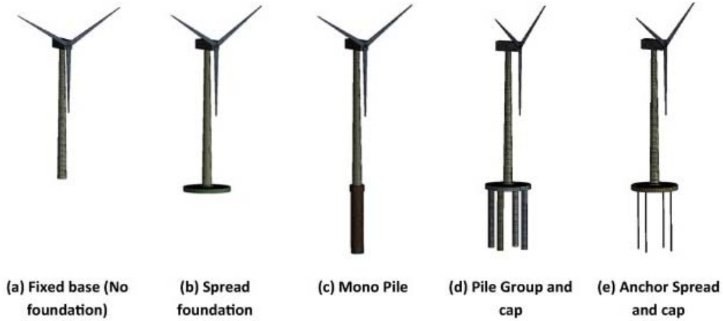
სურათი 3-6 ანძის ფუნდამენტების მაგალითები
