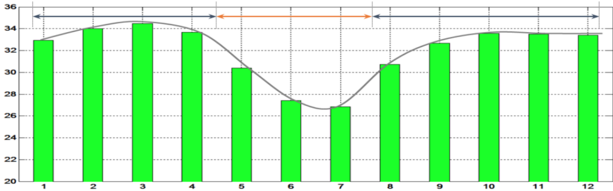
სურათი 3-2 ქეს იმერეთი-1-ის გამომუშავების სეზონურობა, IFC Advisory (აბსცისა - თვეები; ორდინატა - ათასი მეგავატ საათი)
