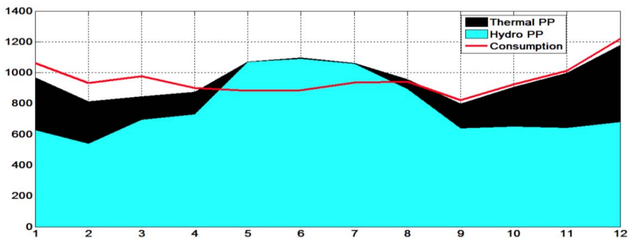
სურათი 3-1 ჯამური ენერჯეტიკული გამომუშავება და გამომუშავების სეზონურობა ენერჯო-წყაროების მიხედვით (შავი - თბოელექტროსადგურები; ცისფერი - ჰესები; წითელი ხაზი - მოხმარების დონეები; (აბსცისა - თვეები; ორდინატა - ათასი მეგავატ საათი)
