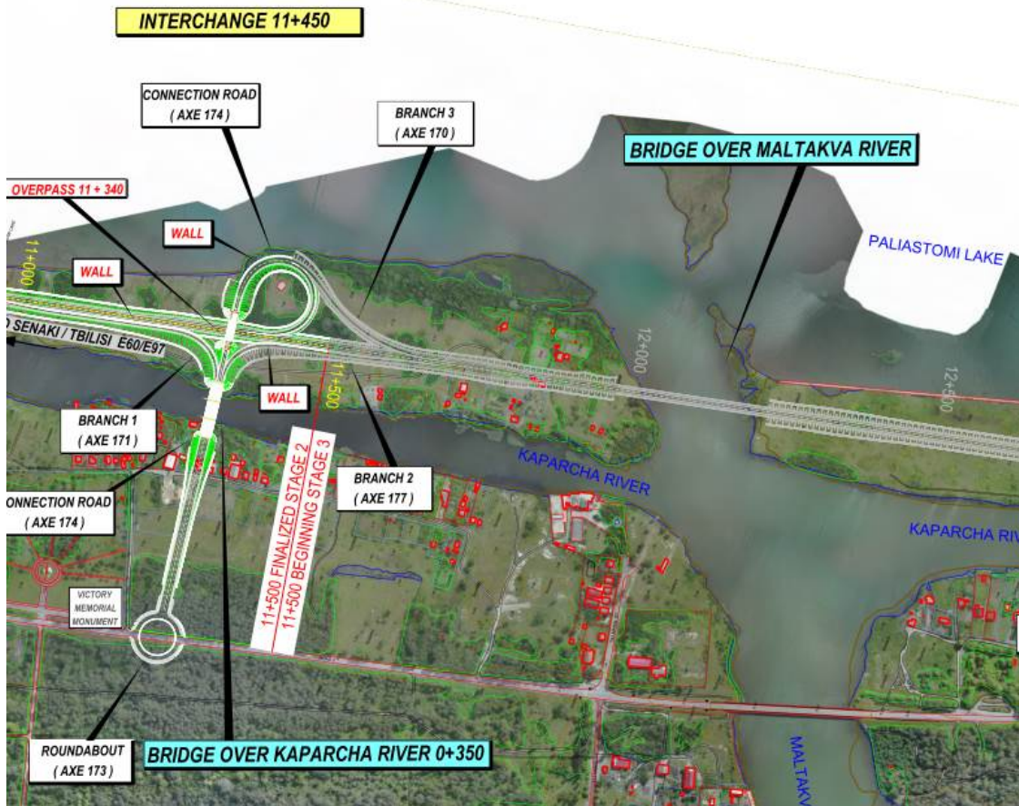
ნახაზი 5. საპროექტო მონაკვეთის ბოლო უბანი
