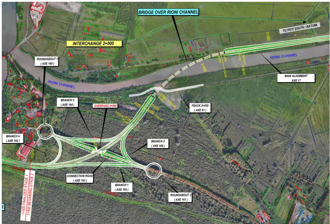
ნახაზი 2. გზის საწყისი უბანი
