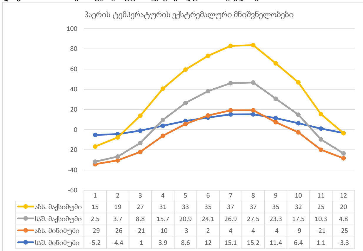
დიაგრამა 3.1.4.1.2 ჰაერის ტემპერატურის ექსტრემალური მნიშვნელობები
