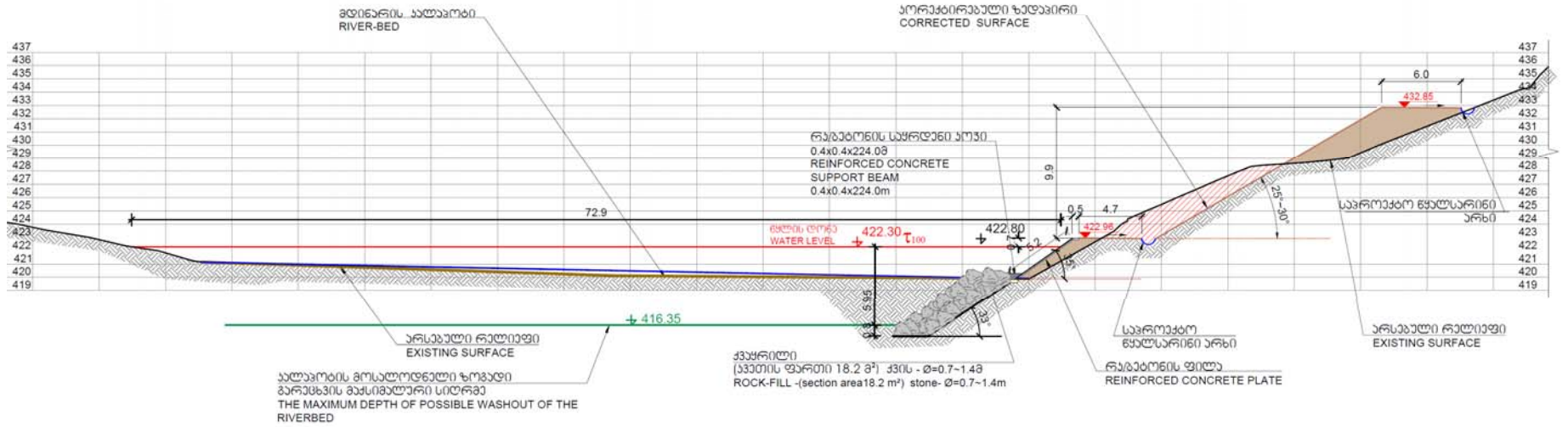
ჭრილი 1-1 SECTION 1-1
