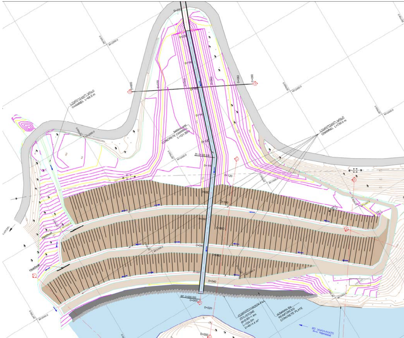
ნახაზი 2.2.1 N6 სანაყაროს გენ-გეგმა
