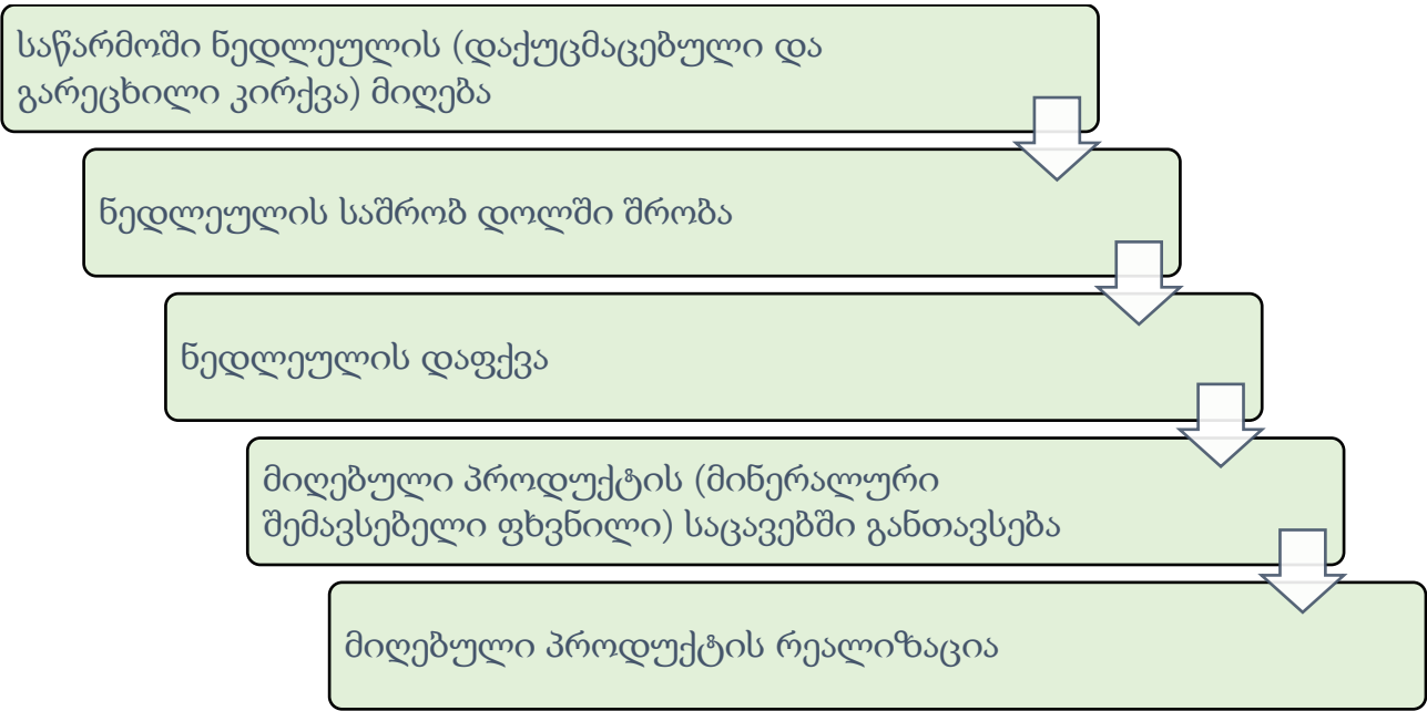
სქემა 2.3.1. - საწარმოს ტექნოლოგიური პროცესების სქემა
