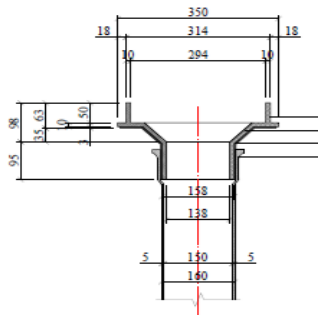
წყალგამწმენდი სისტემა მ. 110
