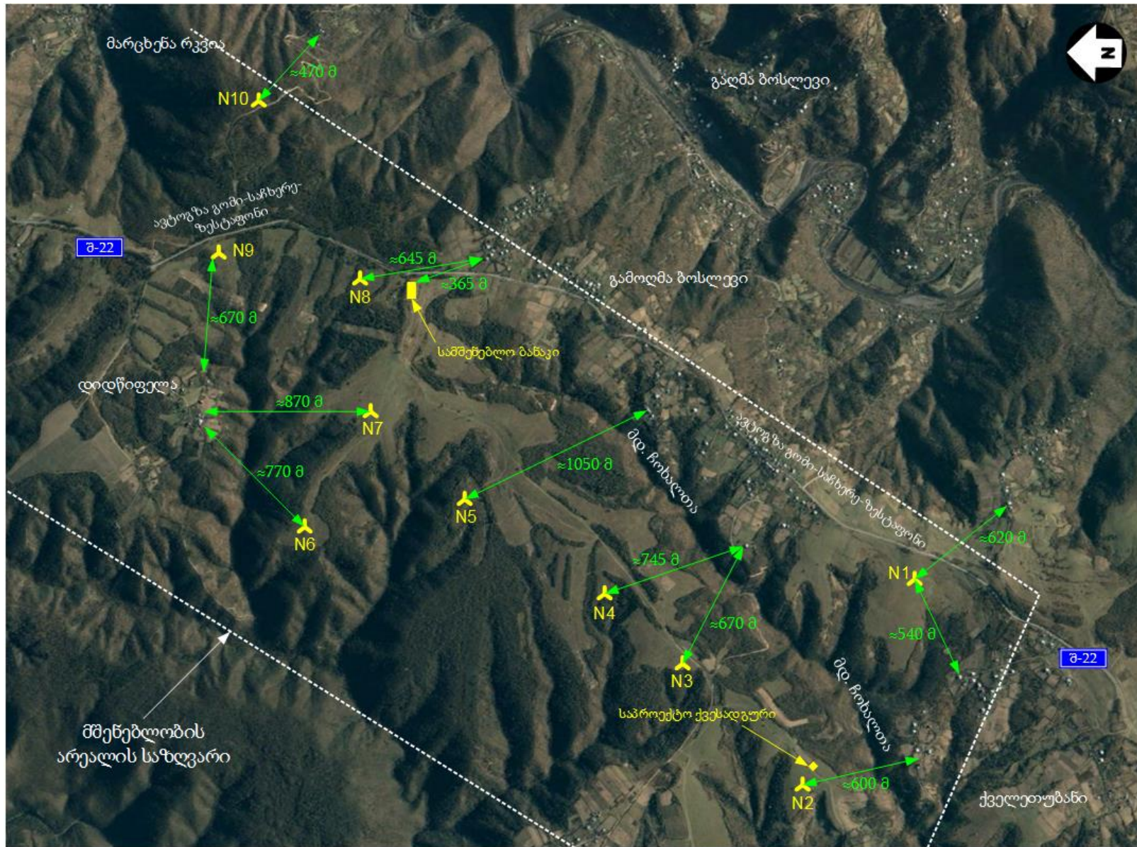
ნახაზი 3.1.1. ქარის ელექტროსადგურის ანძების განლაგების სიტუაციური სქემა
