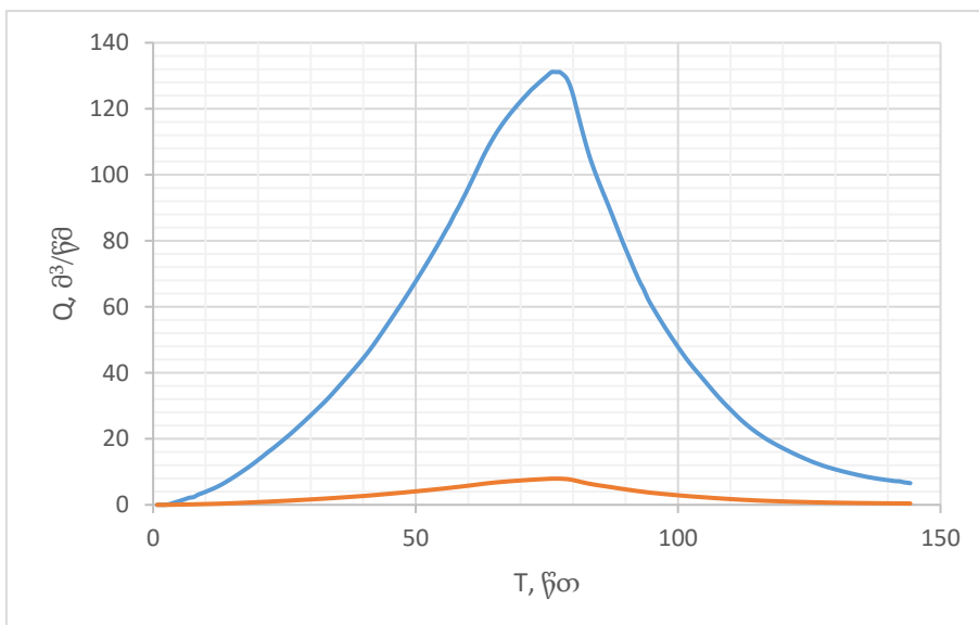
ფიგურა 3.6 მდ. ვახას წყლის 100 წლიანი ხარჯის ჰიდროგრაფი და მყარი ნატანის გრაფიკი
