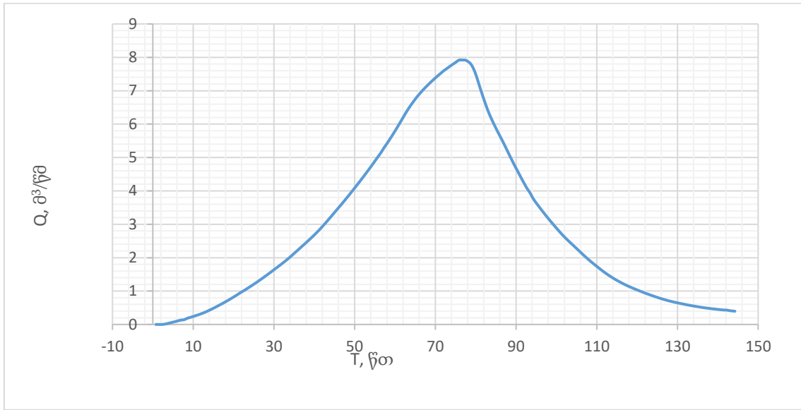
ფიგურა 3.5 მდ. ვახას წყლის ნაკადის მყარი ნატანის გრაფიკი
