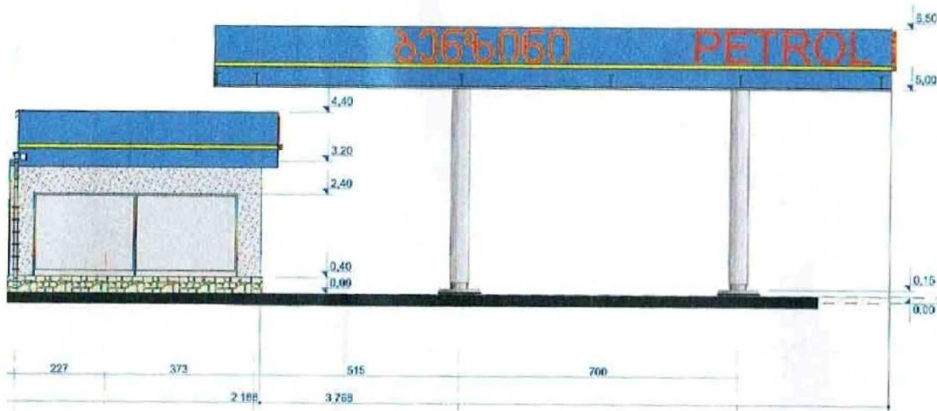
ფასადი ხაზი „ღ-ღ“
