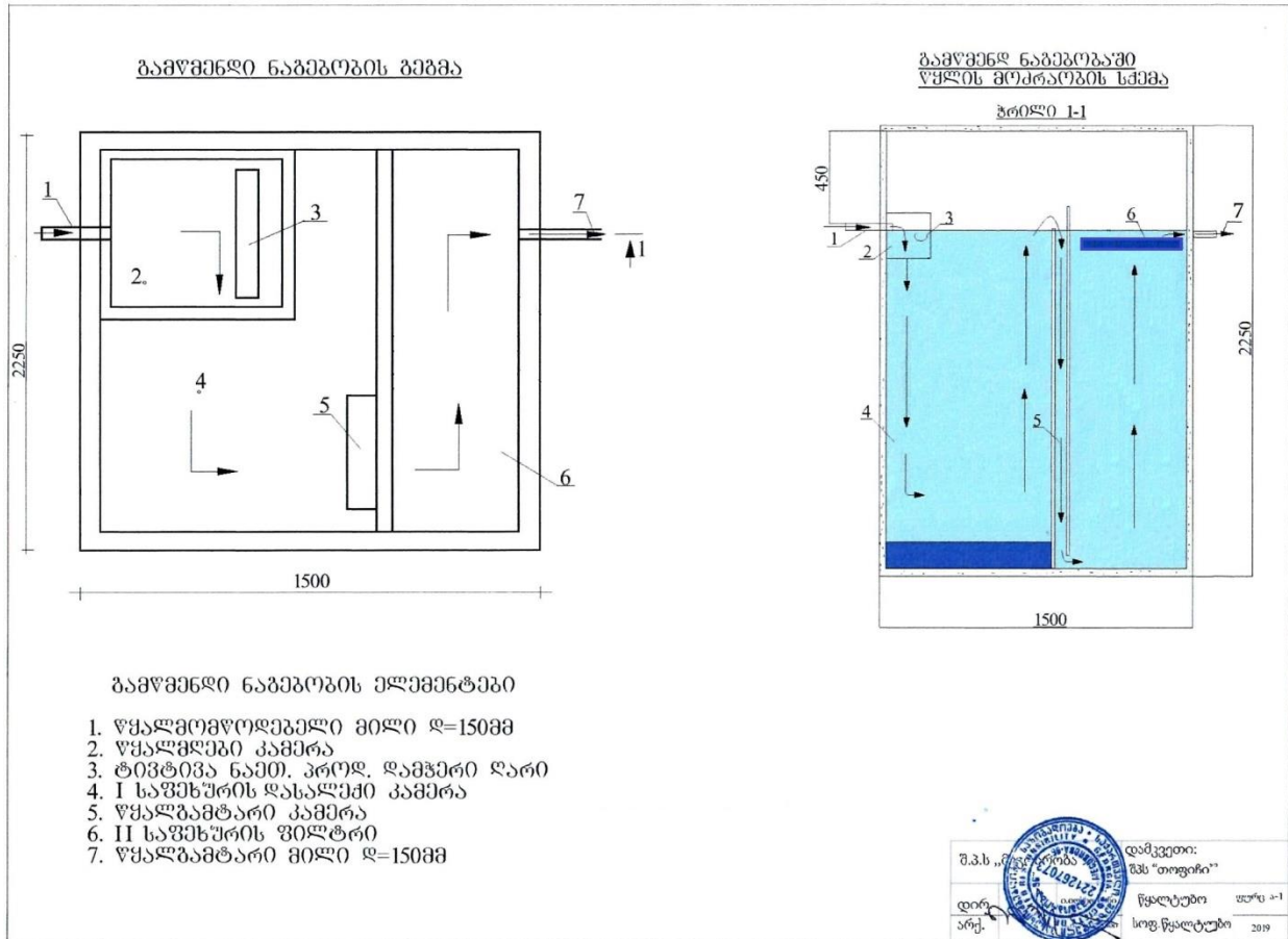
დანართი 4.5. კომპაქტური გამწმენდი ნაგებობა სქემა (ჭრილი და გეგმა)
