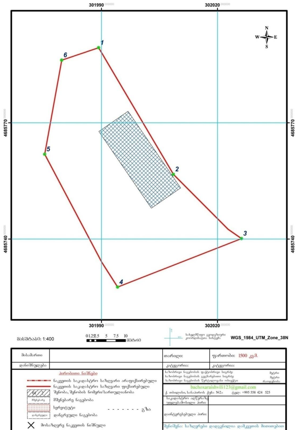
ნახაზი 2.1.1. საკადასტრო აგეგმვითი/აზომვითი ნახაზი
