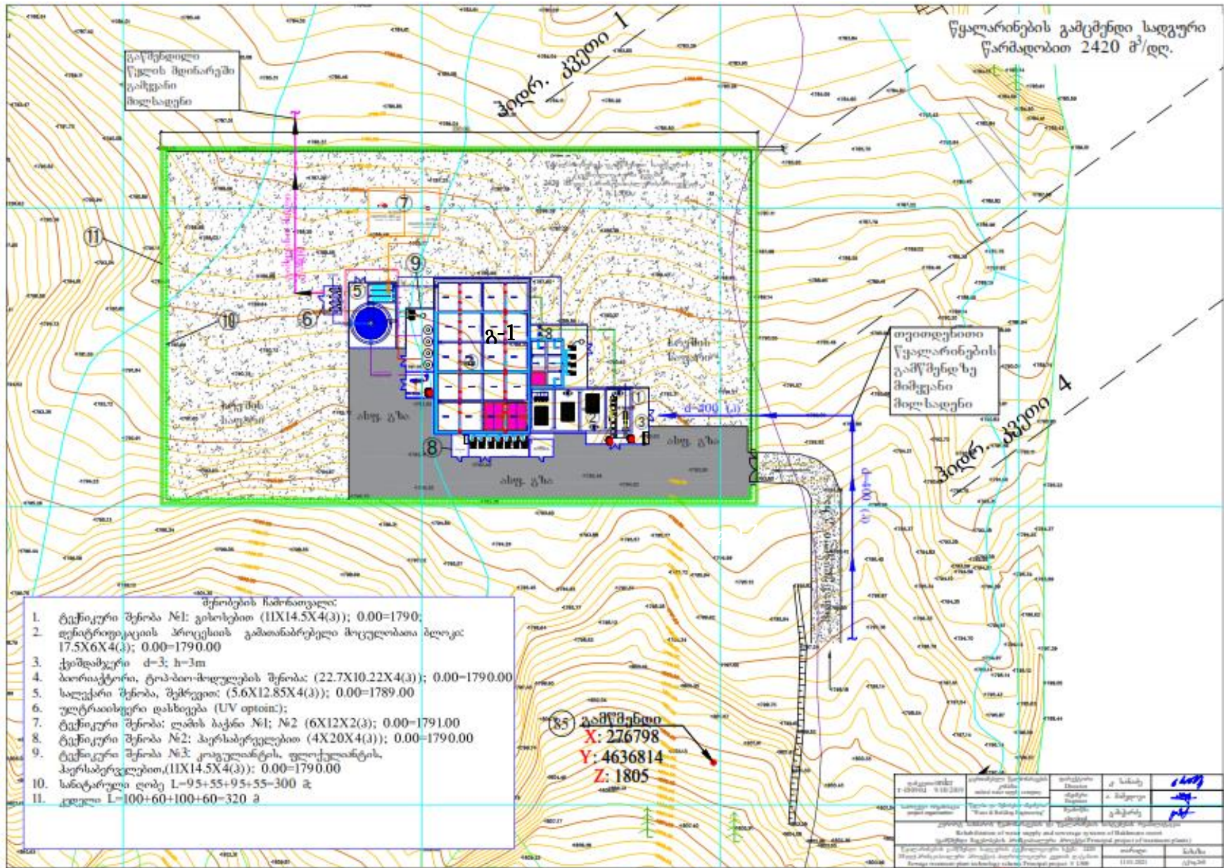
დან. 1 გამწმენდი ნაგებობის (წარმადობით 2400 მ 3 /დღ.ტ.) გენ-გეგმა გაფრქვევის წყაროების ჩვენებით
