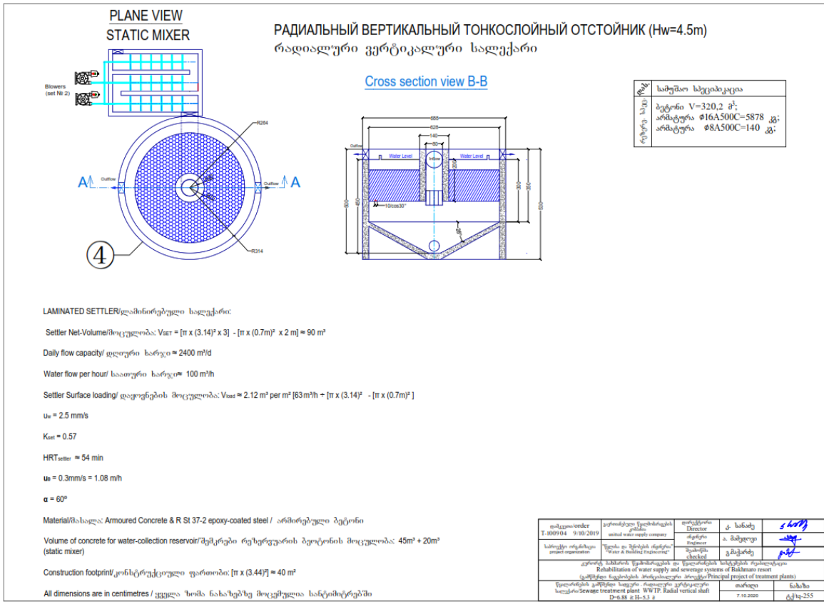
სურ. 4.7.3 - რადიალური ვერტიკალური სალექარი
