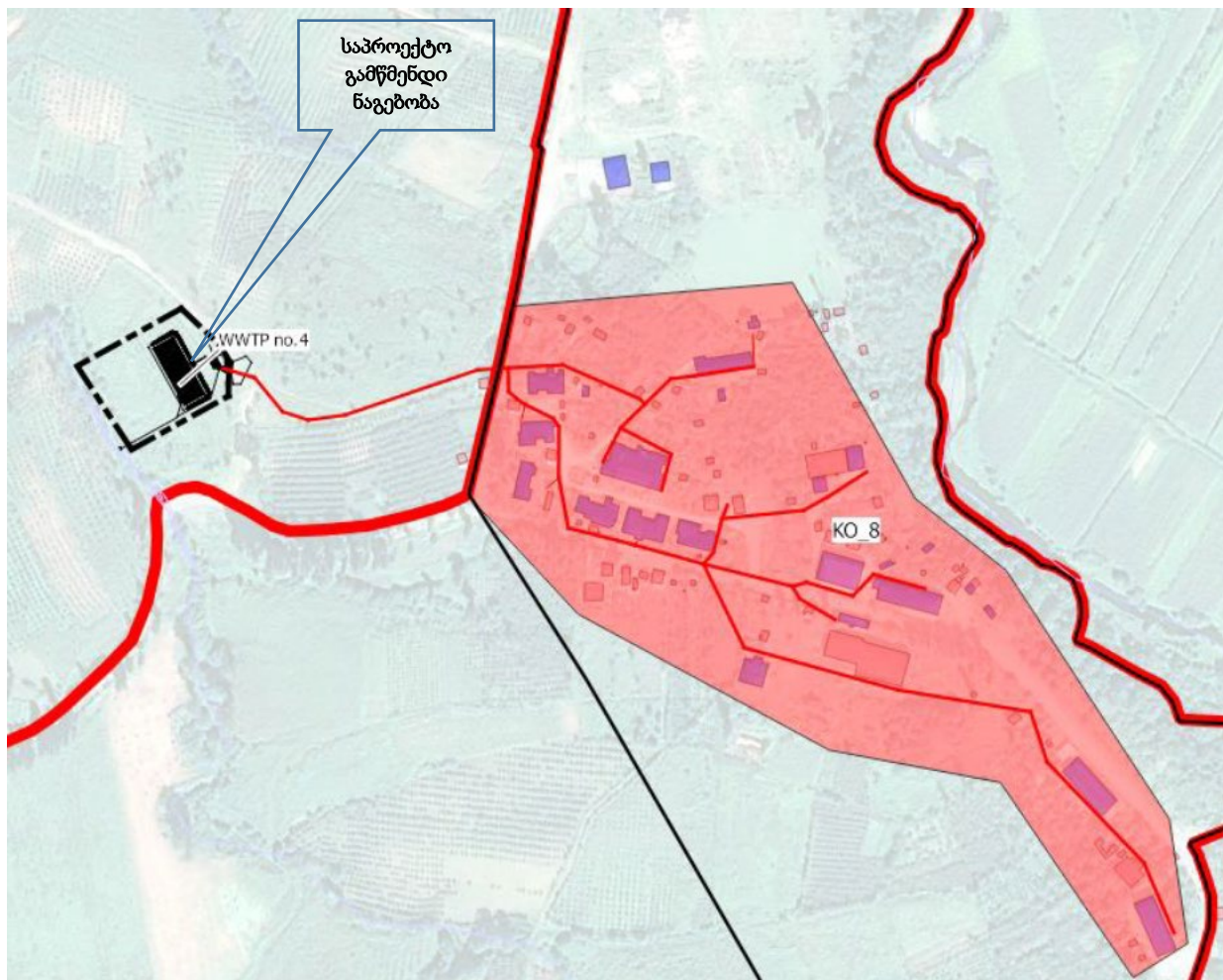
ნახაზი 3.6.1. საპროექტო საკანალიზაციო ქსელის არეალი (მონიშნულია ვარდისფრად)
