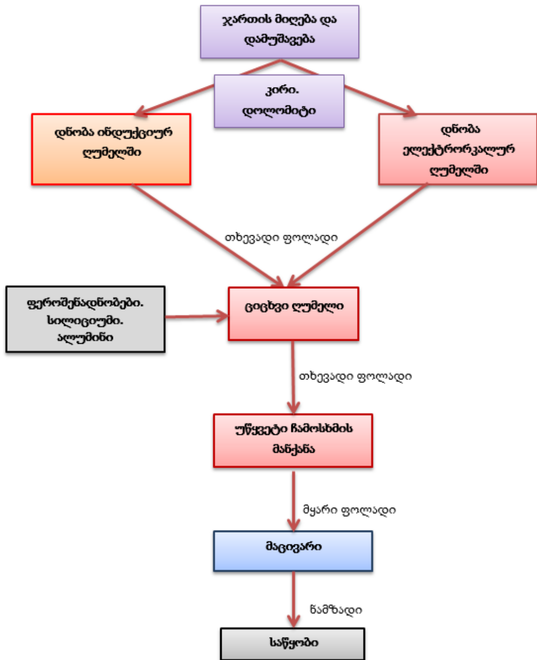
ნახაზი 5.1. ტექნოლოგიური სქემა
