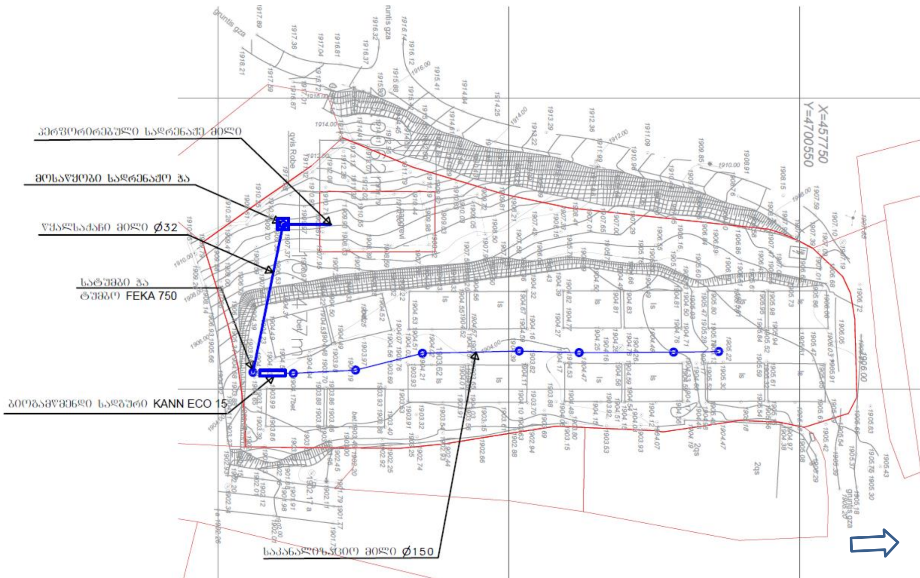
ნახაზი 2.2.1. კოტეჯების გეგმა წყლარინების სქემის დატანით
