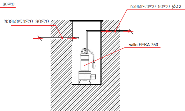
სატუმბო ჭა
