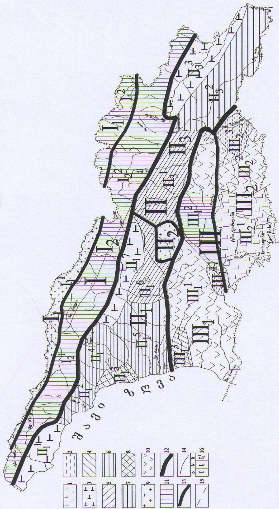
ნახ. 7. საქართველოს აბრეგეოლოგიური დარღობების და აბრეგეოქიმიური ზონალურობის სქემატური რუკა
