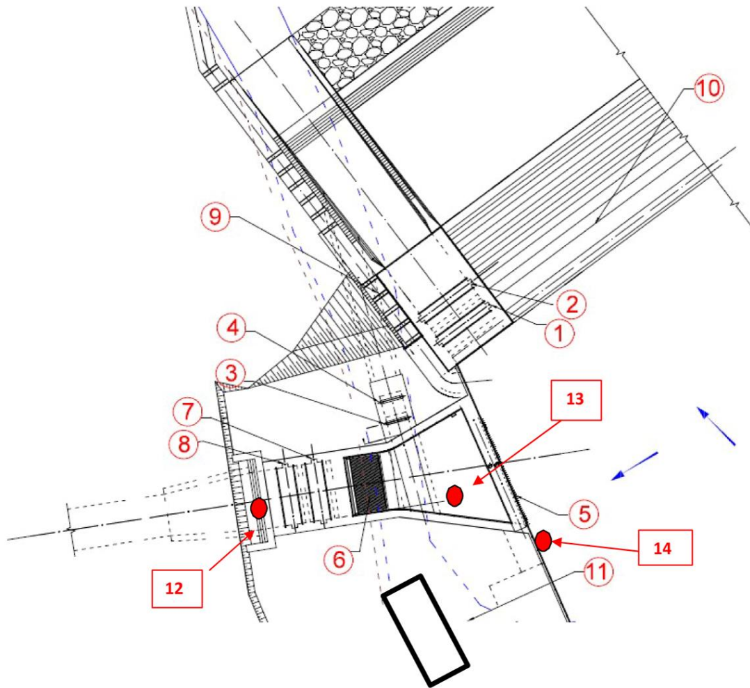
ნახაზი 2. სათავე კვანძის გეგმა
