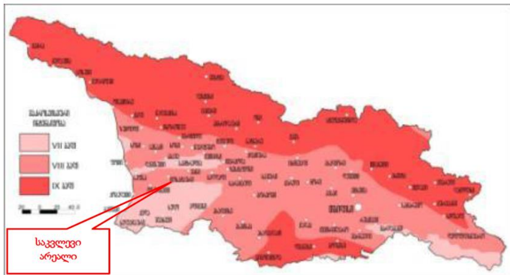
ნახაზი 6. საქართველოს სეისმური დარაიონების რუკა
