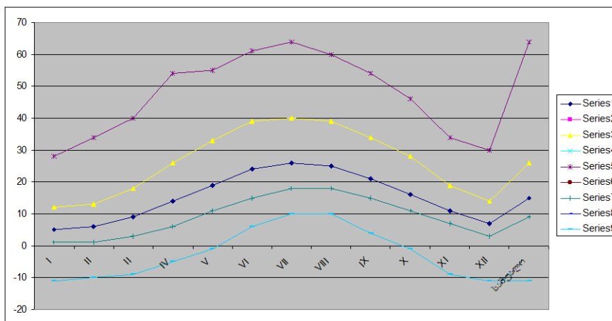
ნახაზი 2.1.3.6. ნიადაგის ზედაპირის საშუალო თვიური, მაქსიმალური და მინიმალური ტემპერატურა
