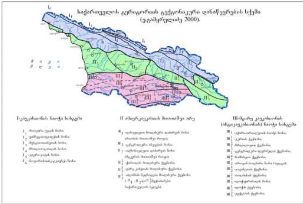
რუკა. 6. საქართველოს ტერიტორიის ტექტონიკური დანაწევრების სქემა
