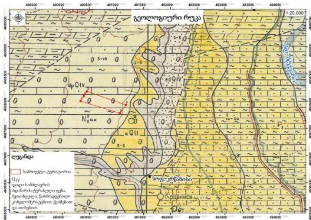
რუკა. 7. გეოლოგიური აგებულება (საფუძველი 1:25 000 საინჟინრო-გეოლოგიური დანაწევრების რუკა, 1981 წ.)
