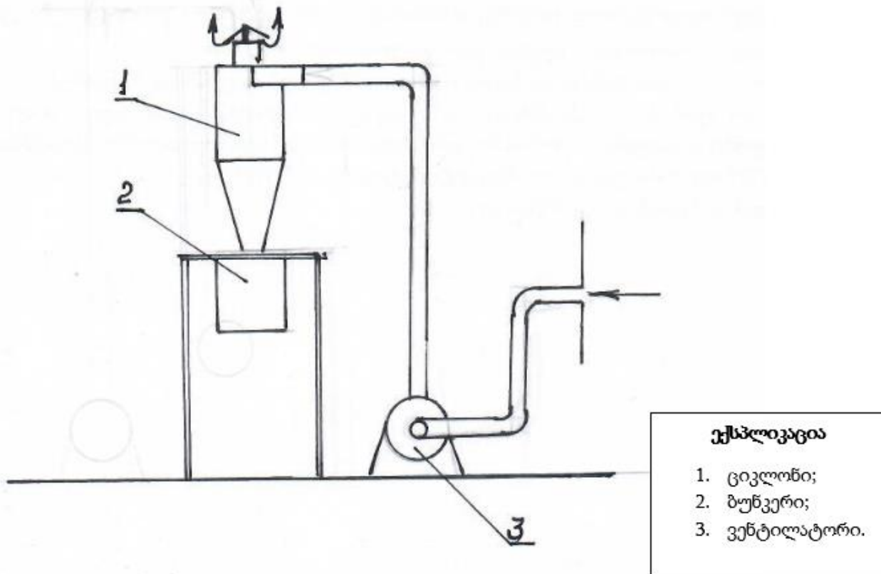
ნახაზი 3.6.
