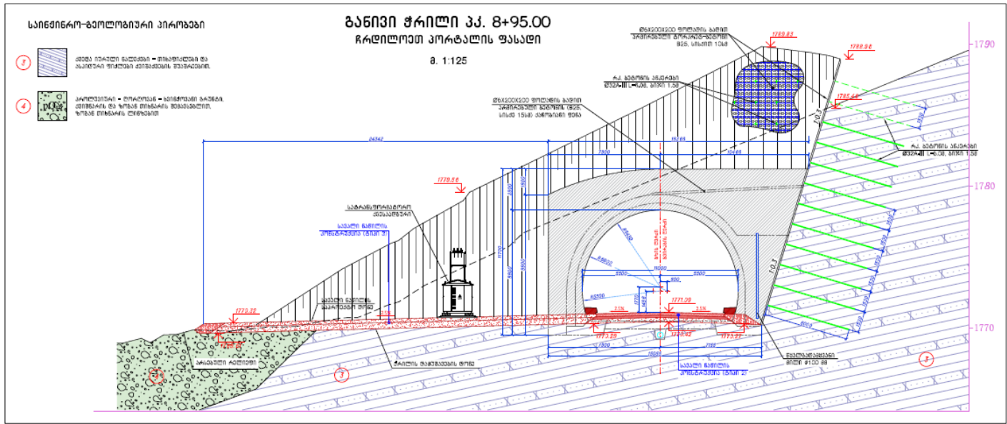
ნახაზი 2.3.3.2. ჩრდილოეთ პორტალის ფასადი
